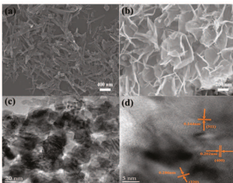
Figure 3. (a) The SEM images of \text{Co}_3\text{O}_4 , (b) \text{Co}_3\text{O}_4/\text{N-HNMK-3} . (c) TEM and (d) HRTEM images of \text{Co}_3\text{O}_4/\text{N-HNMK-3} .
