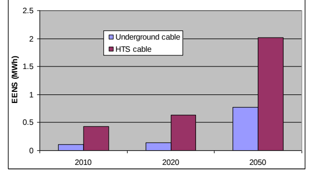
Fig.5. Comparison of EENS
