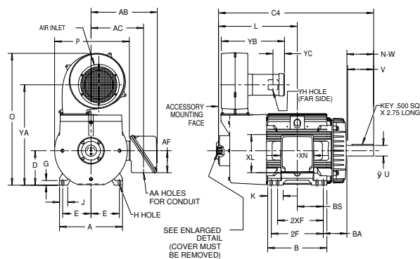
364-5013 Frame (TEBC)
