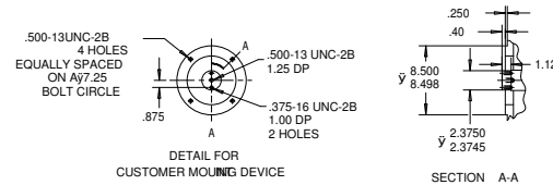
364-5013 Frame (TEBC)
