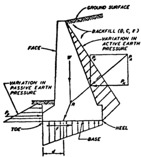
A. GRAVITY
