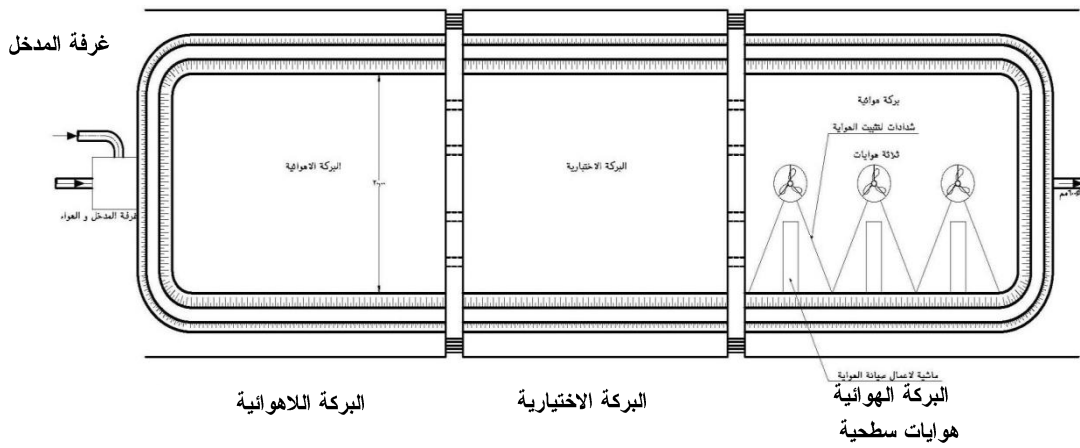
شكل رقم (13) شكل تخطيطي لنظام المعالجة باستخدام برك الأكسدة الموهوة ميكانيكيا
