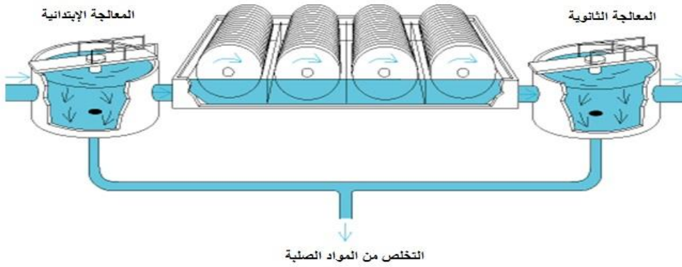
شكل رقم (2) وحدات معالجة مياه
