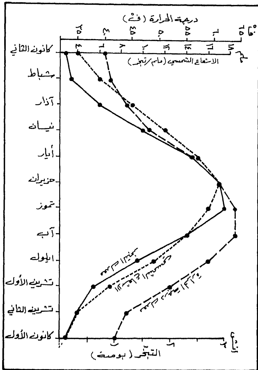
شكل (16) منحنى المعدل الشهري للتبخر الكلي
