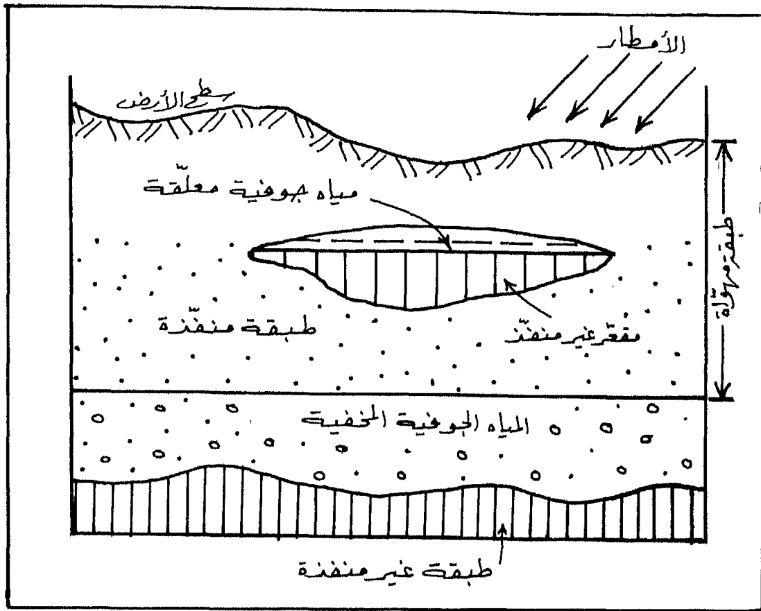
شكل (37) الطبقات المائية الجوفية المعلقة
