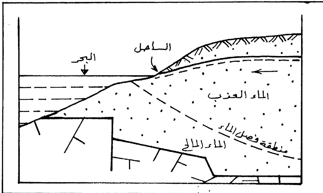
شكل (41) المياه الجوفية الكارستية
