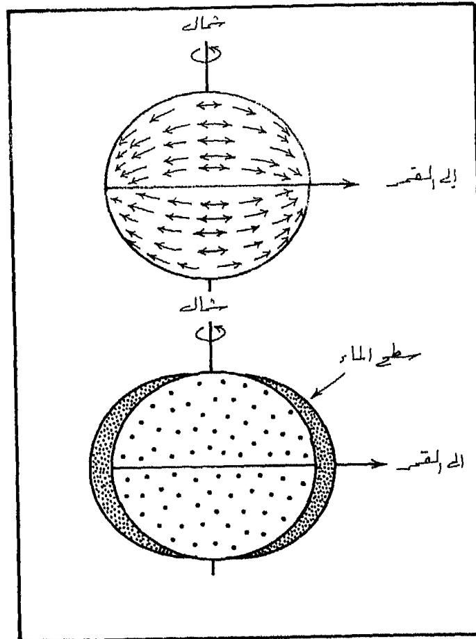
شكل (56) اختلاف المد حسب موقع الساحل بالنسبة لخطوط العرض
