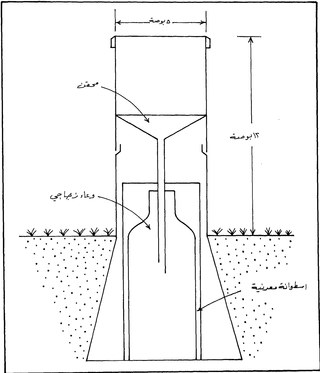
شكل (9) جهاز قياس المطر (5 بوصة) النموذج البريطاني
