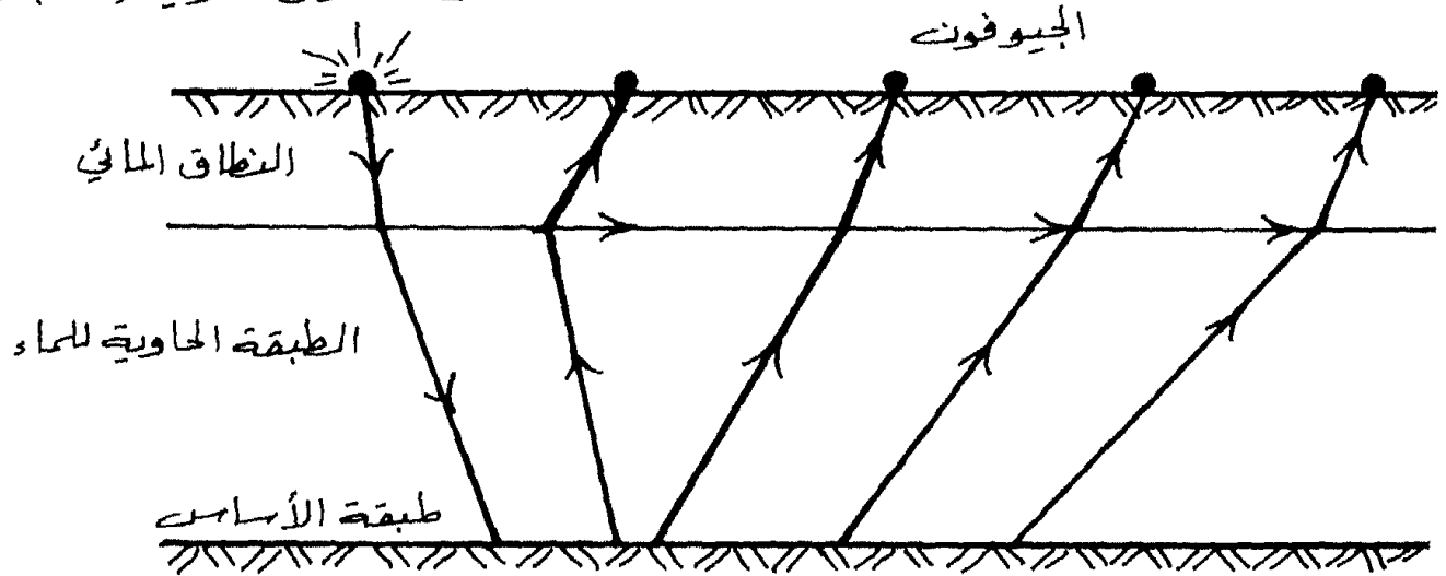
شكل (45) طريقة الانكسار السيزمية لمعرفة عمق الماء الجوفي
