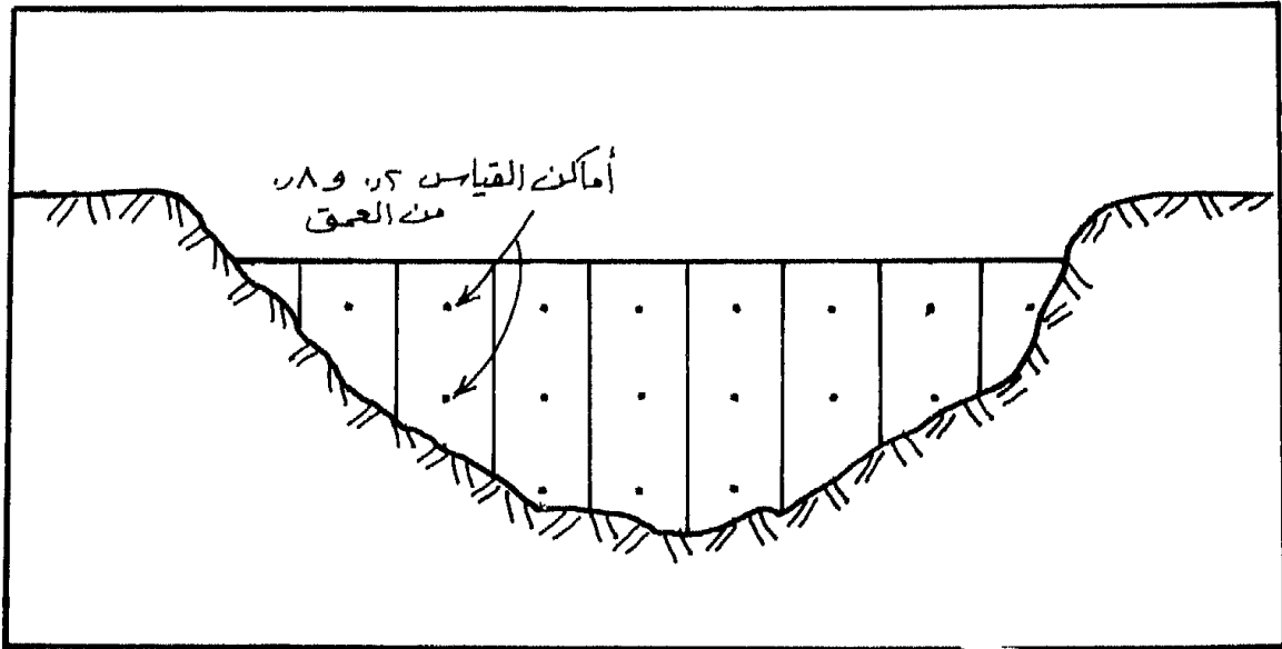
شكل (24) أماكن قياس سرعة الماء في الجرى
