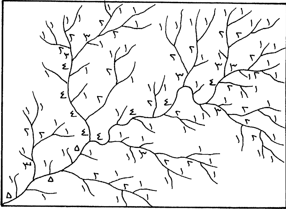
شكل (4) الرتب النهرية
