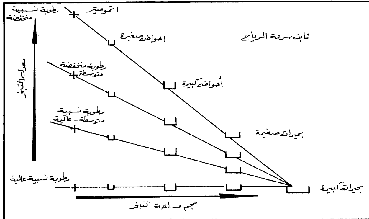
شكل (18) معدل التبخر من مسطحات مائية صغيرة الحجم واسعة المساحة
