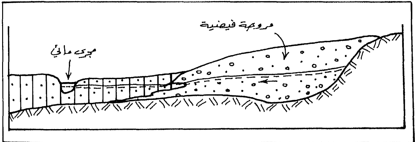
شكل (40) المياه الجوفية تحت المراوح المعلقة
