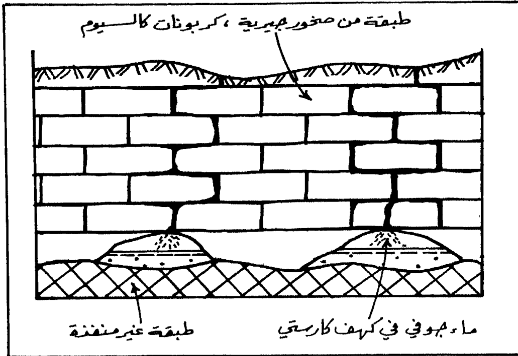
شكل (41) المياه الجوفية الكارستية
