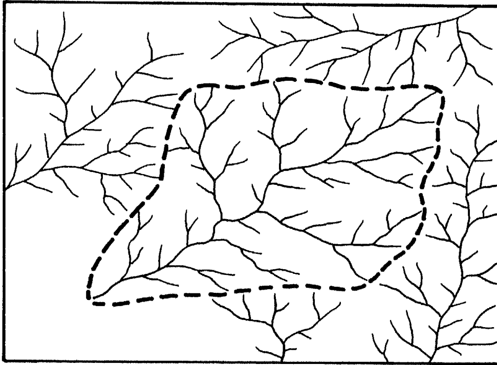
شكل (3) تحديد الحوض النهرى
