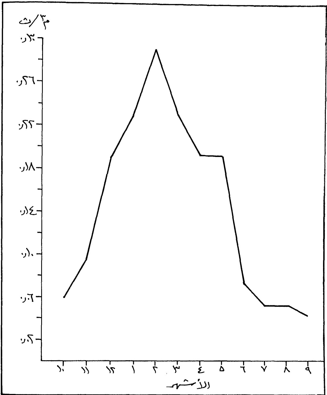
شكل (28) تصريف الأساس
