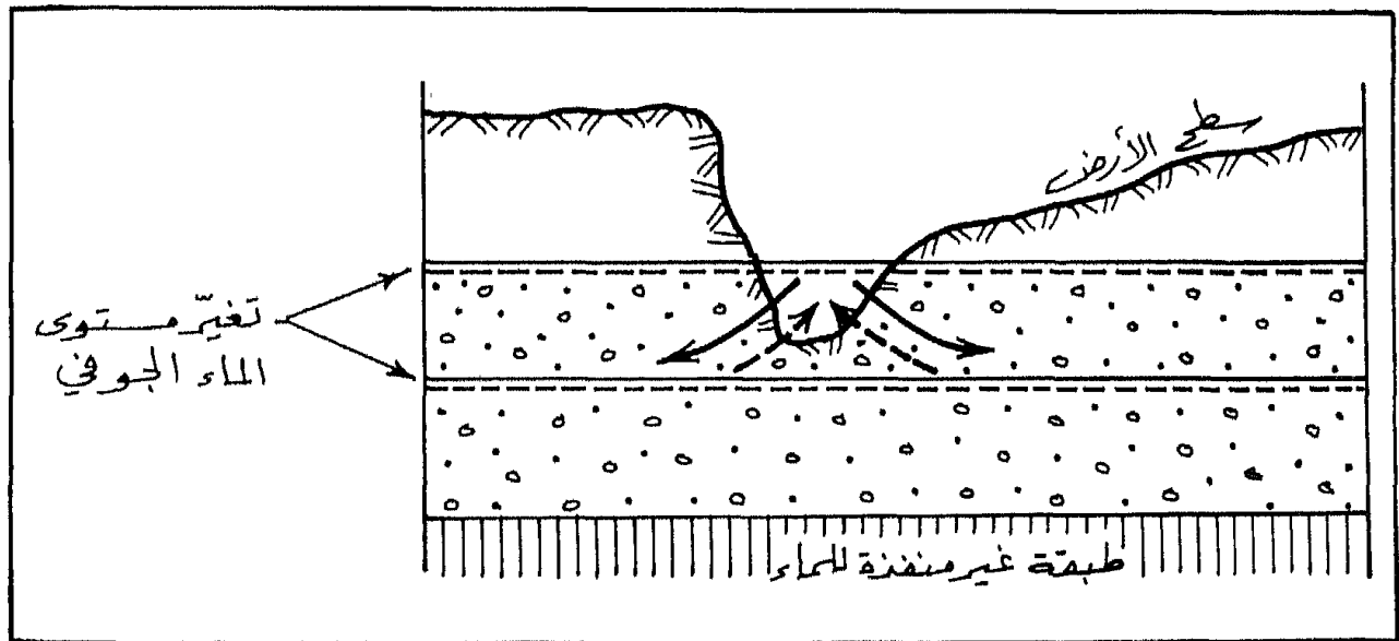
شكل (37) الطبقات المائية الجوفية المعلقة
