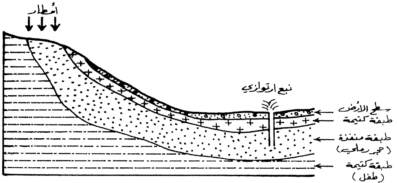
شكل (47) التدفق الارتوازي
