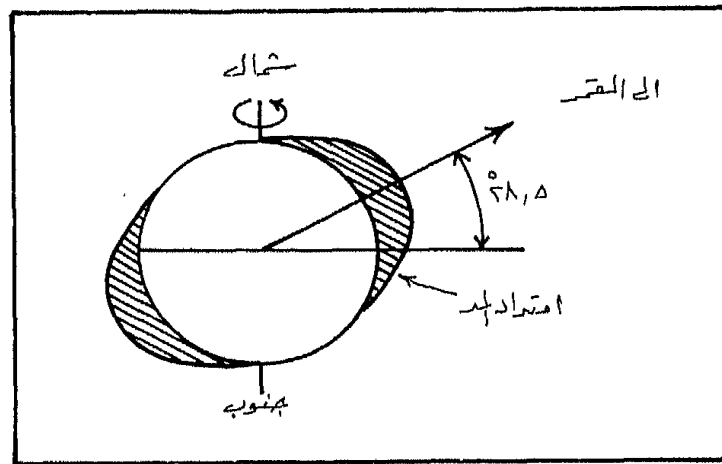
شكل (58) تأثير ميل محور الأرض وميل محور القمر على تفاوت المد والجزر
