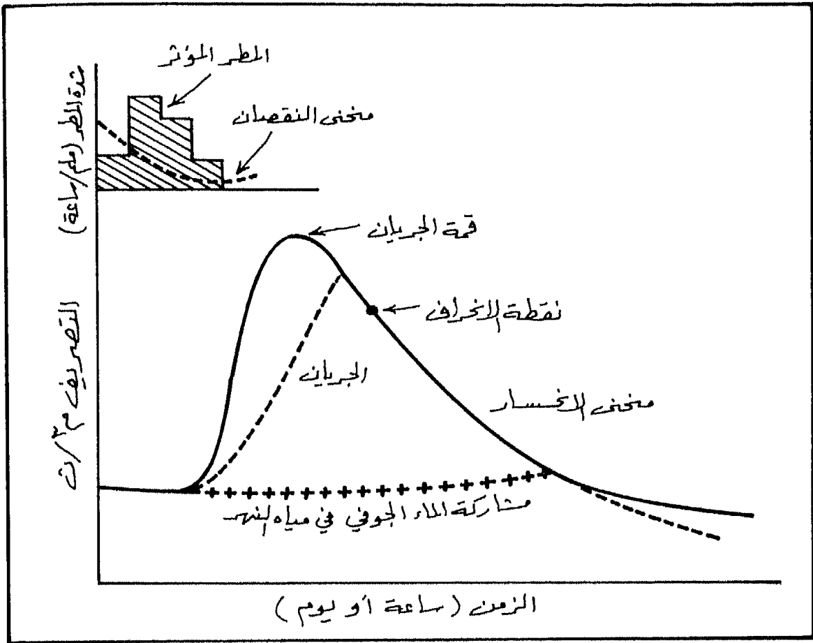
شكل (26) عناصر منحنى الجريان المائي
