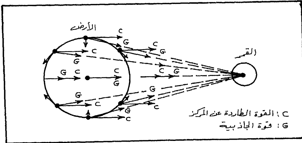
شكل (55) العلاقة بين المد والجزر ومركز القمر
