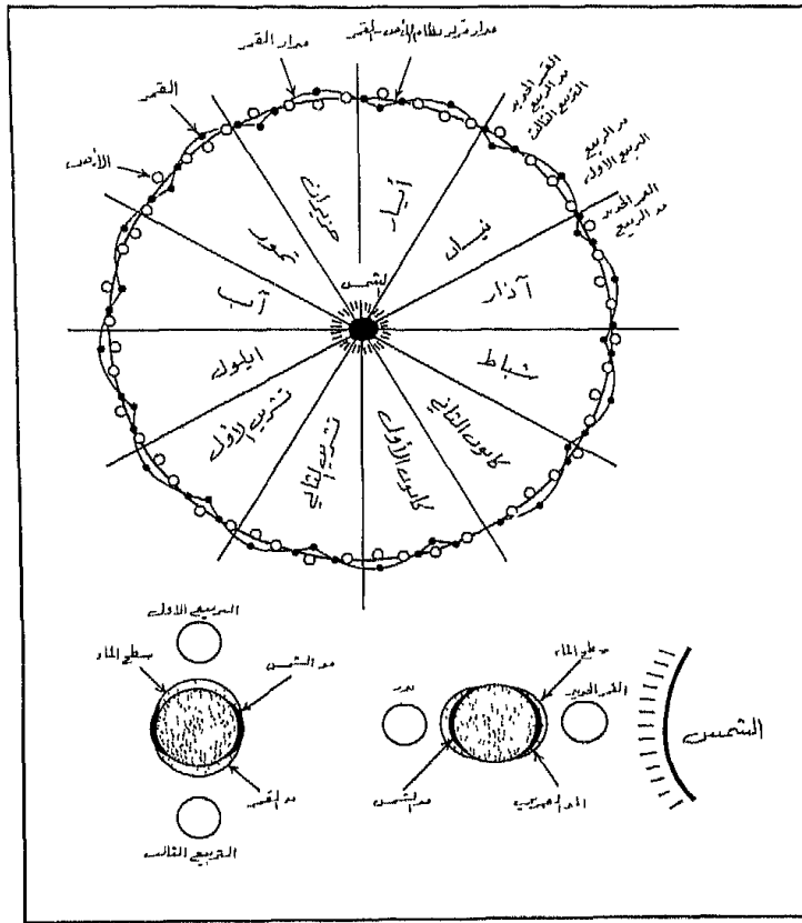
شكل (57) العلاقة بين المد ومنازل القمر
