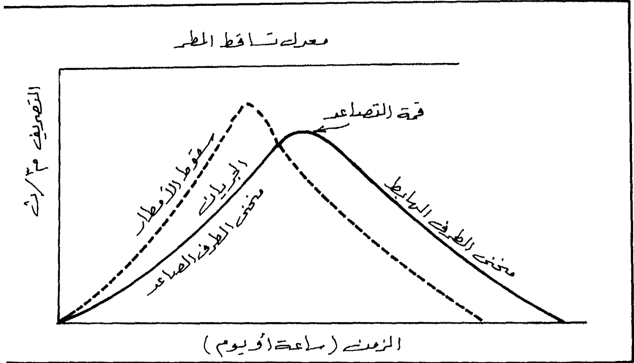
شكل (27) مكونات منحنى الجريان المائي
