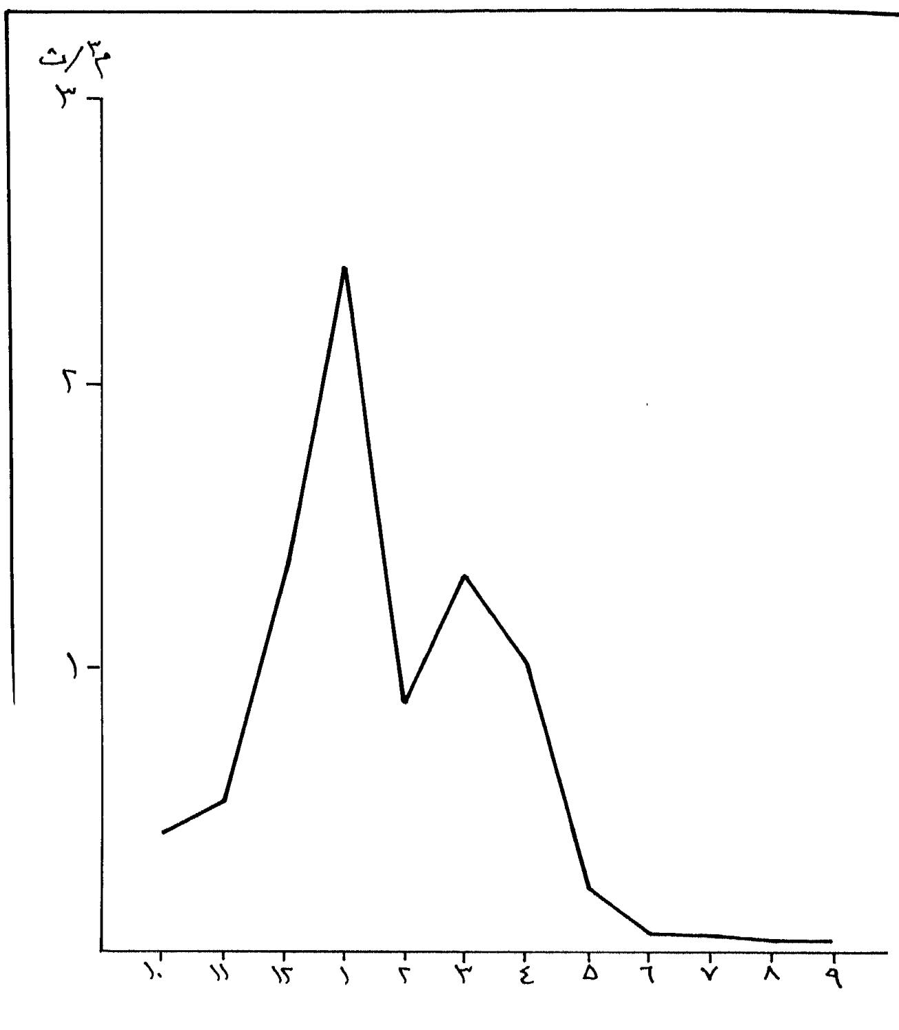
شكل (29) التصريف اليومي
