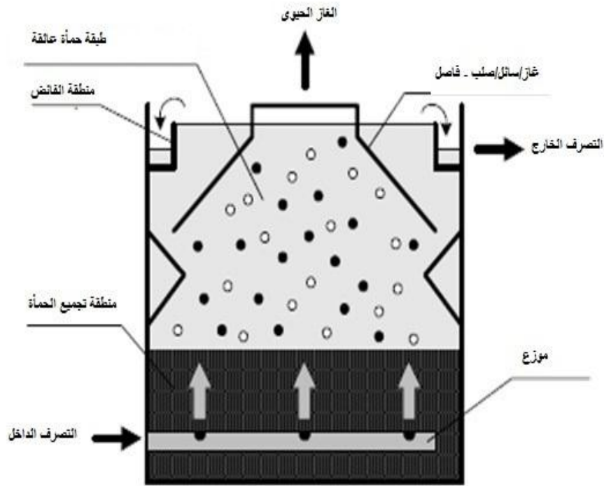
شكل رقم (18) تفاصيل حوض المعالجة اللاهوائية من أسفل لأعلى (UASB)
