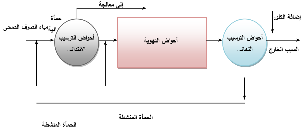
شكل رقم (٤) نظام المعالجة بالحمأة المنشطة التقليدية
