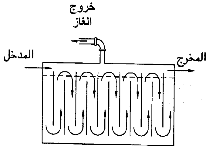
شكل رقم (15) حوض التفاعل البيولوجي اللاهوائي ذو حواجز تمر به المياه لأعلى وأسفل وأفقيا
