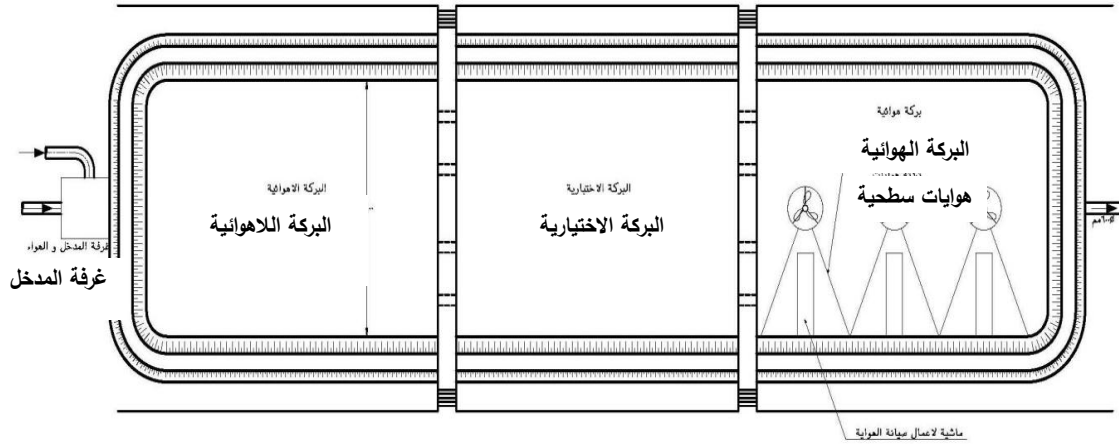
شكل رقم (١٣) شكل تخطيطي لنظام المعالجة باستخدام برك الأكسدة المهباه ميكانيكيا
