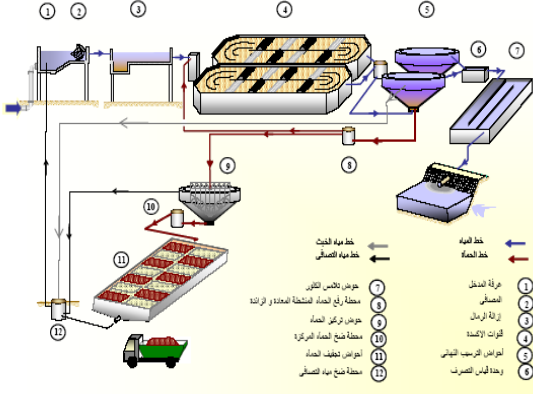
شكل رقم ٦ مخطط لمحطة معالجة الصرف الصحي نظام تهويه ممتدة
