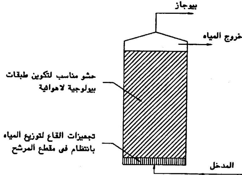
شكل رقم (١٦) تفاصيل المرشح اللاهوائي الرأسي (الميل لأعلى)
