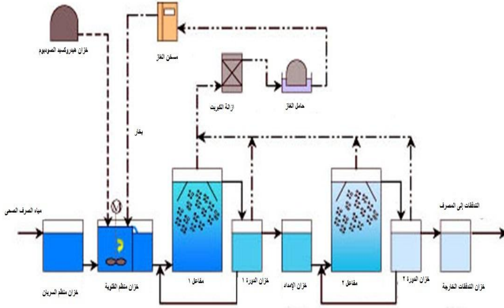
شكل رقم (19) مخطط لمحطة معالجة الصرف الصحي باستخدام الأحواض اللاهوائية من أسفل إلى أعلى (UASB)
