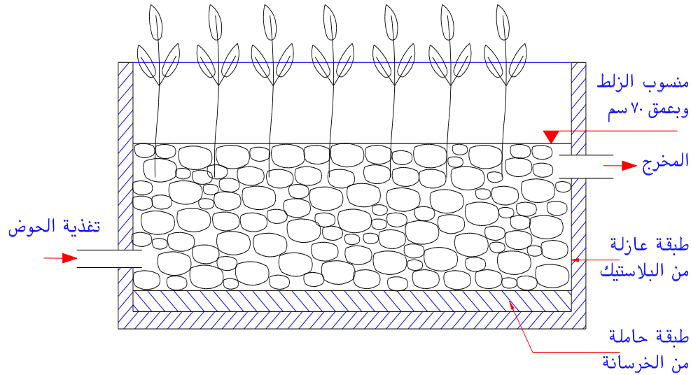
شكل رقم ٢٢ نظام التدفق تحت السطحى
