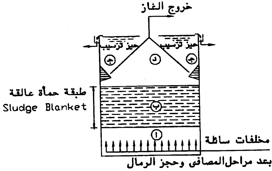
شكل رقم (17) طريقة لاهوائية تتجه فيها المياه لأعلى خلال طبقة حمأة
