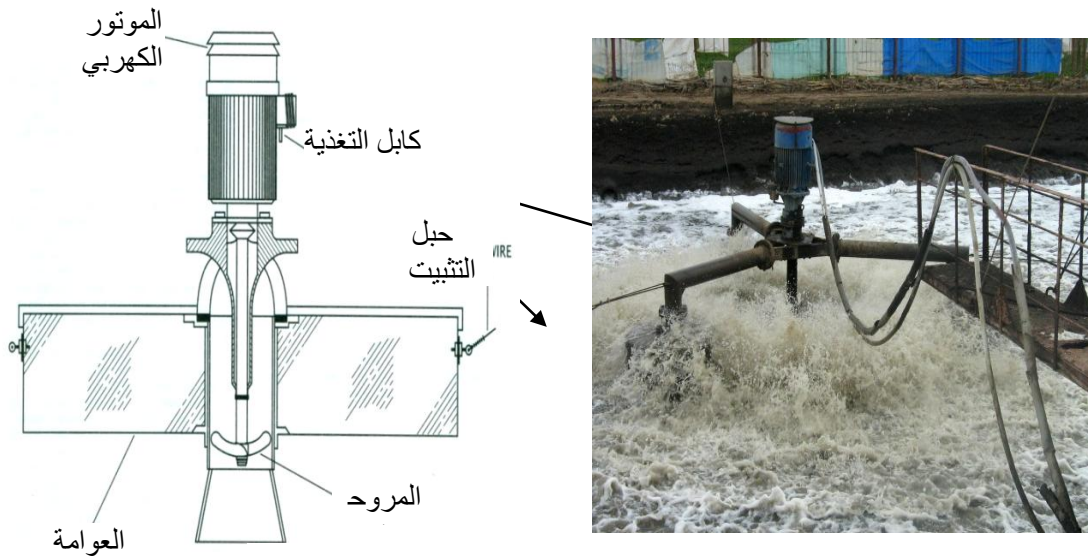
صورة رقم (١٤) الهوايات المستخدمة في تهوية برك الأكسدة المهواة
