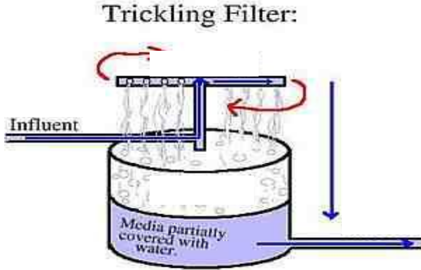
شكل رقم (٤-٢) يوضح قطاعاً لمكونات المرشح الزلطي
