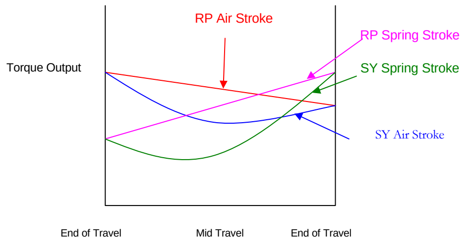
Figure 4: SA actuator torque curve
