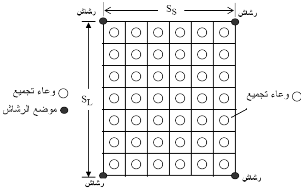
شكل (٣-٤). تجربة قياس عمق الماء للرشاشات بتوزيع العلب في المساحة التي يخدمها الرشاش
