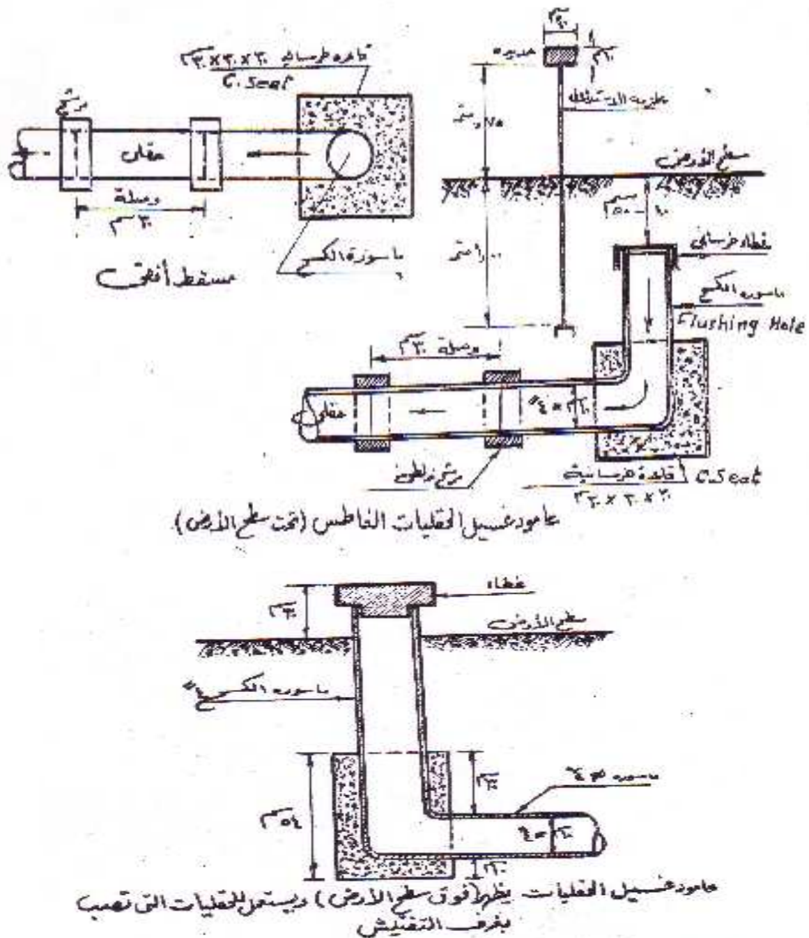
شكل ( ٤-٩ ) مواسير الكسح للغسيل المتواجدة تحت سطح الأرض والمتواجدة أعلى سطح الأرض.
