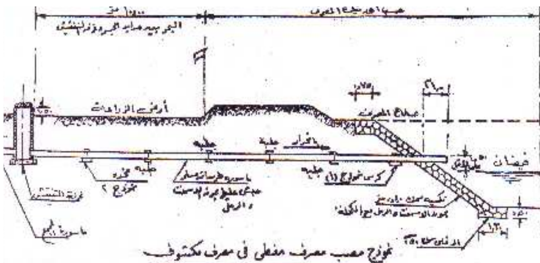
شكل (٤-١٥) نموذج لمصب مصرف مغطى في مصرف مكشوف.
