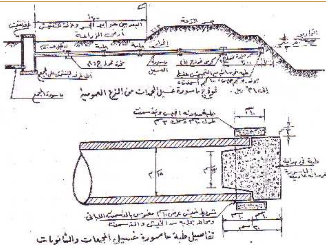
شكل (٤-١١) نموذج لماسورة غسيل المجمعات وكذلك تفاصيل طبقة هذه المواسير.
