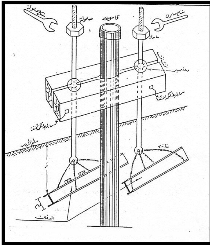
شكل (١-١٤) طريقة ربط الفتائل والدفان مع ماسورة البئر
