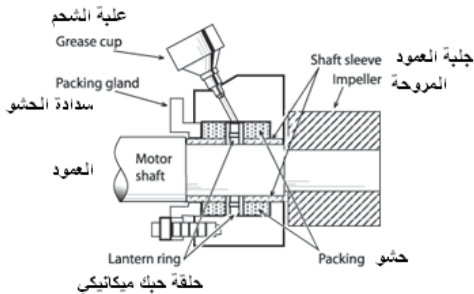
شكل (٣-٧). رسم تخطيطي يبين حشو المضخات
