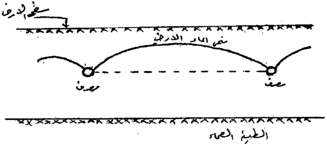
شكل (٧-٤) مصرفين جوفيين (مصارف مغطاة)
