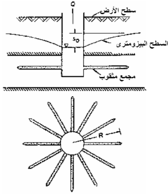
شكل (١-١٢) بئر التجمع القطري
