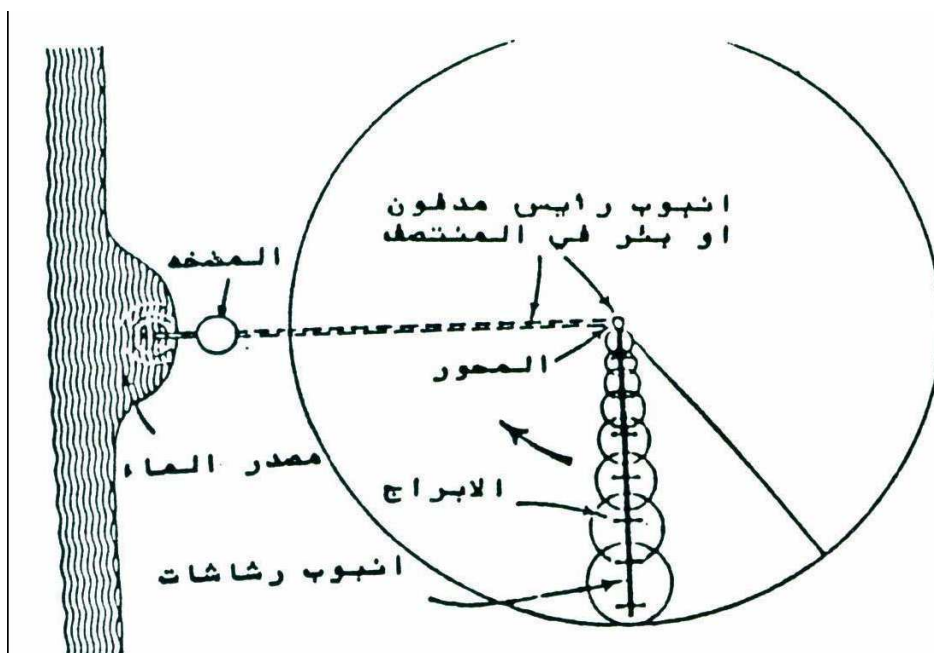
شكل (٢-٢٤) وصف النظام المحوري
