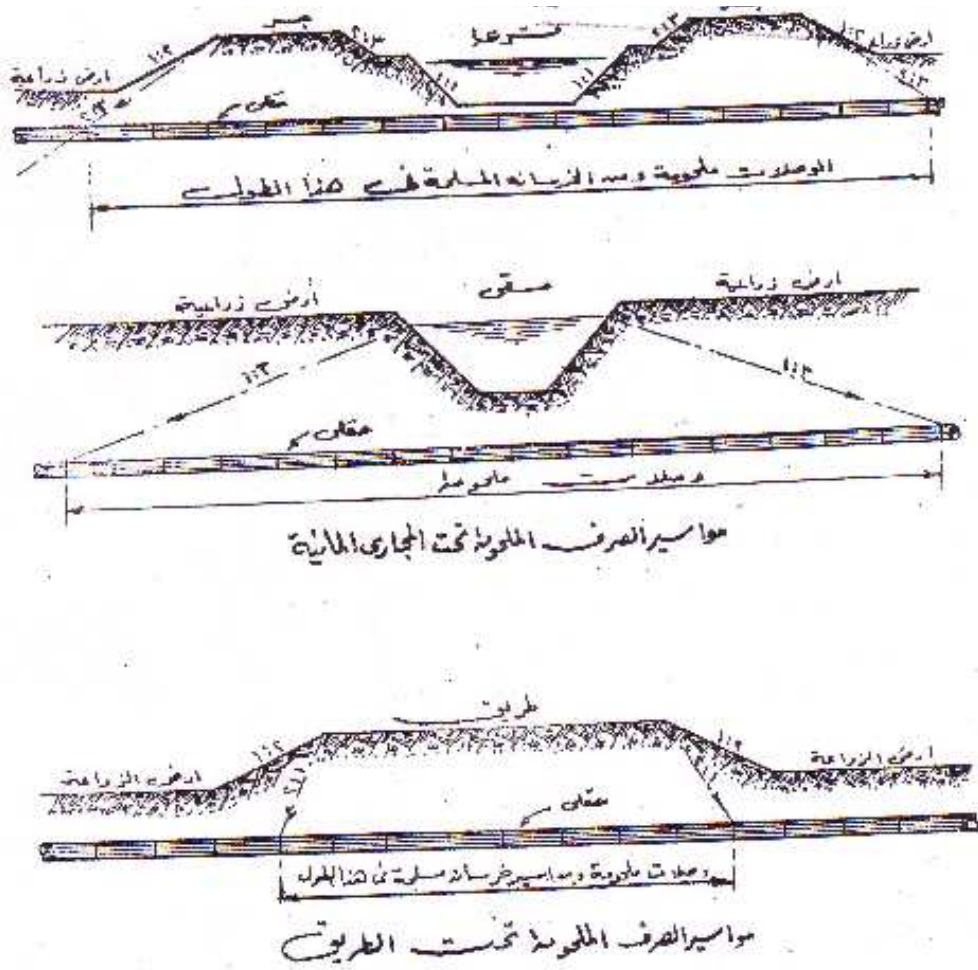
شكل (١٧-٤) وصلات المواسير الملحومة سواء على طول أورنيك الترعة أو تحت المجارى المائية أو تحت الطريق.
