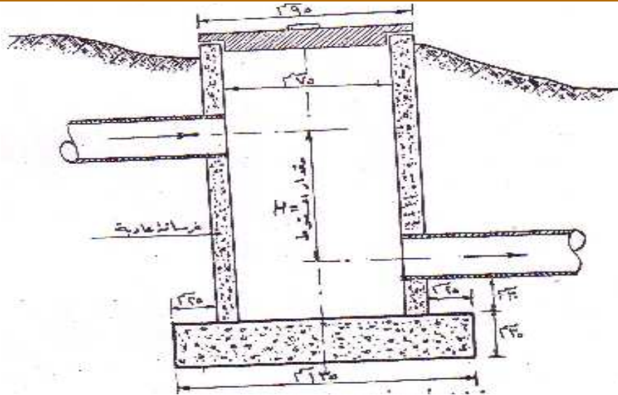
شكل (٤-١٤) قطاع رأسي بأحد المساقط (Falls)
