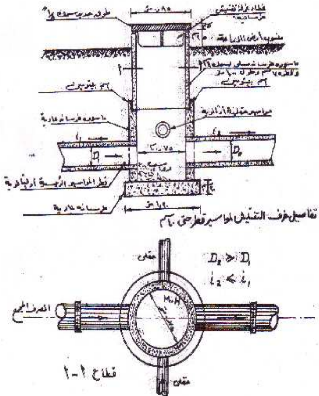
شكل (٤-١٢). تفاصيل غرف التفريش عند نقط الاتصال بين مواسير الحقليات مع المجمعات لمواسير قطر حتى ٤٠ سم.
