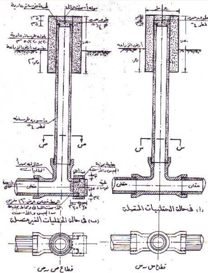
شكل ( ١٠-٤ ) نماذج لأعمدة الاستدلال في حالة الحقلية المتصلة وفي حالة الحقلية الغير
