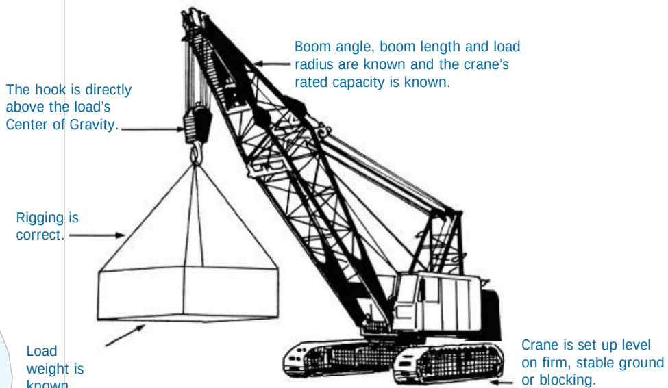
Fig. 18 17.5.3. Crawler Crane
