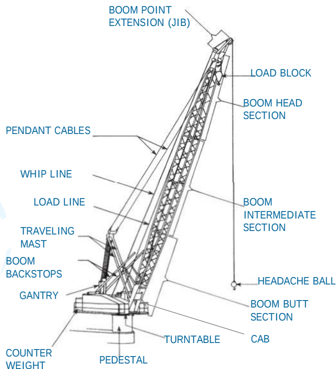
Fig. 19 17.5.4. Offshore Crane
