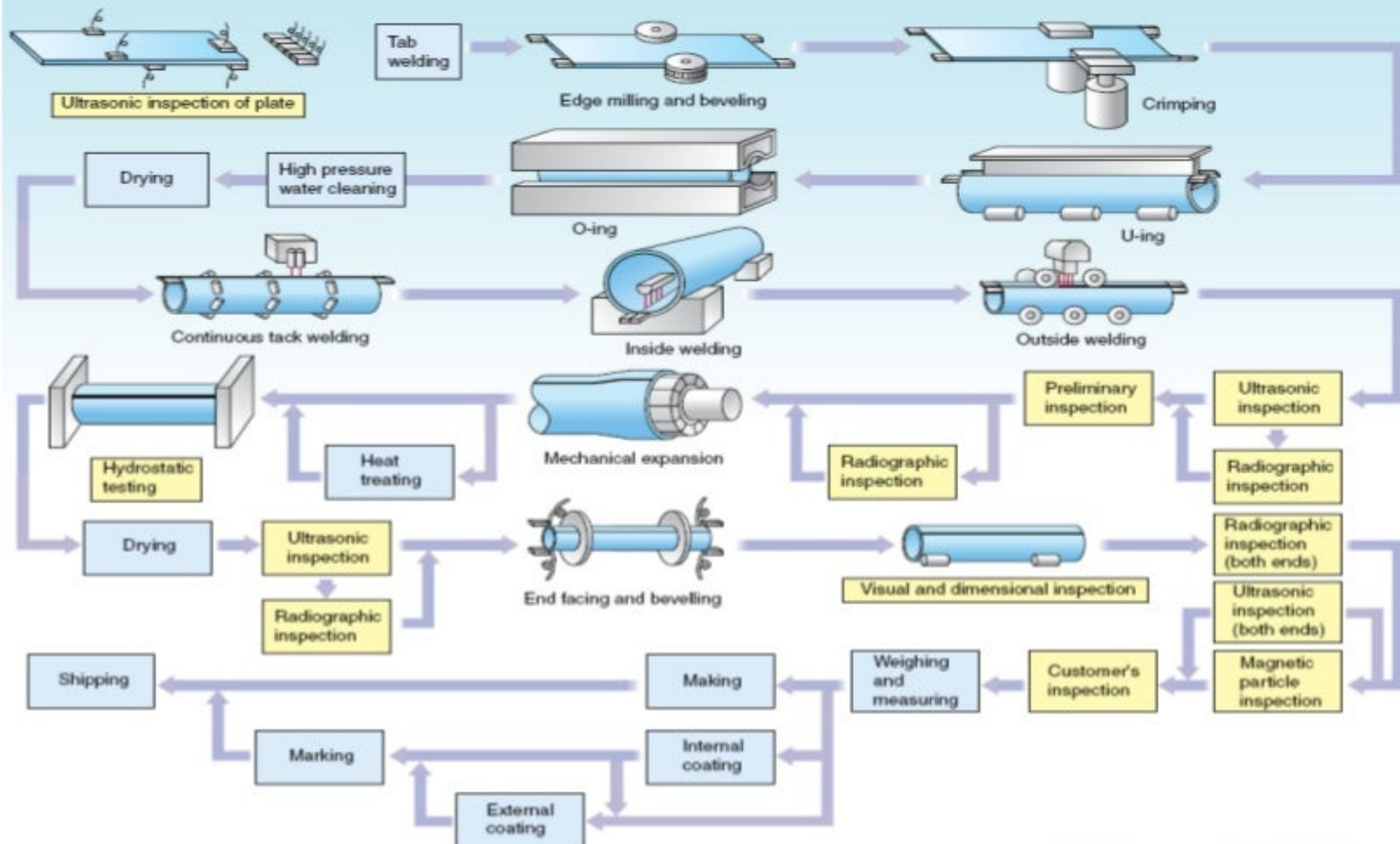
Fukuyama UOE Pipe
