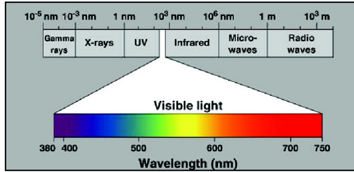
شكل يوضح الطول الموجي للأشعة فوق البنفسجية
