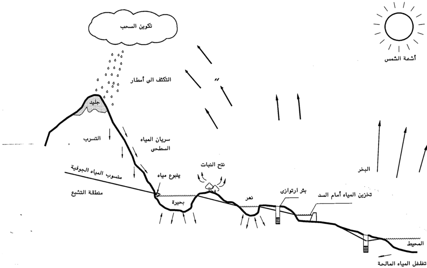
شكل رقم (١-٢) الدورة الهيدرولوجية
