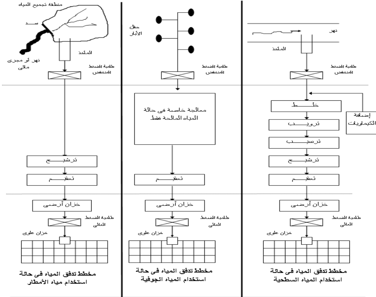
مخطط نظام الإمداد بمياه الشرب من المصادر المختلفة
