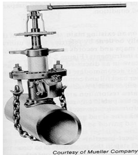
ماكينة ثقب المواسير
