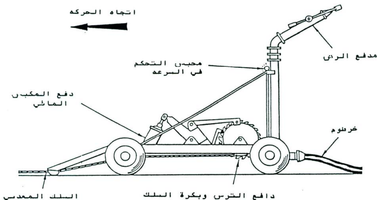
شكل (٣ - ١) مكونات النظام المدفعي المسحوب بسلك
