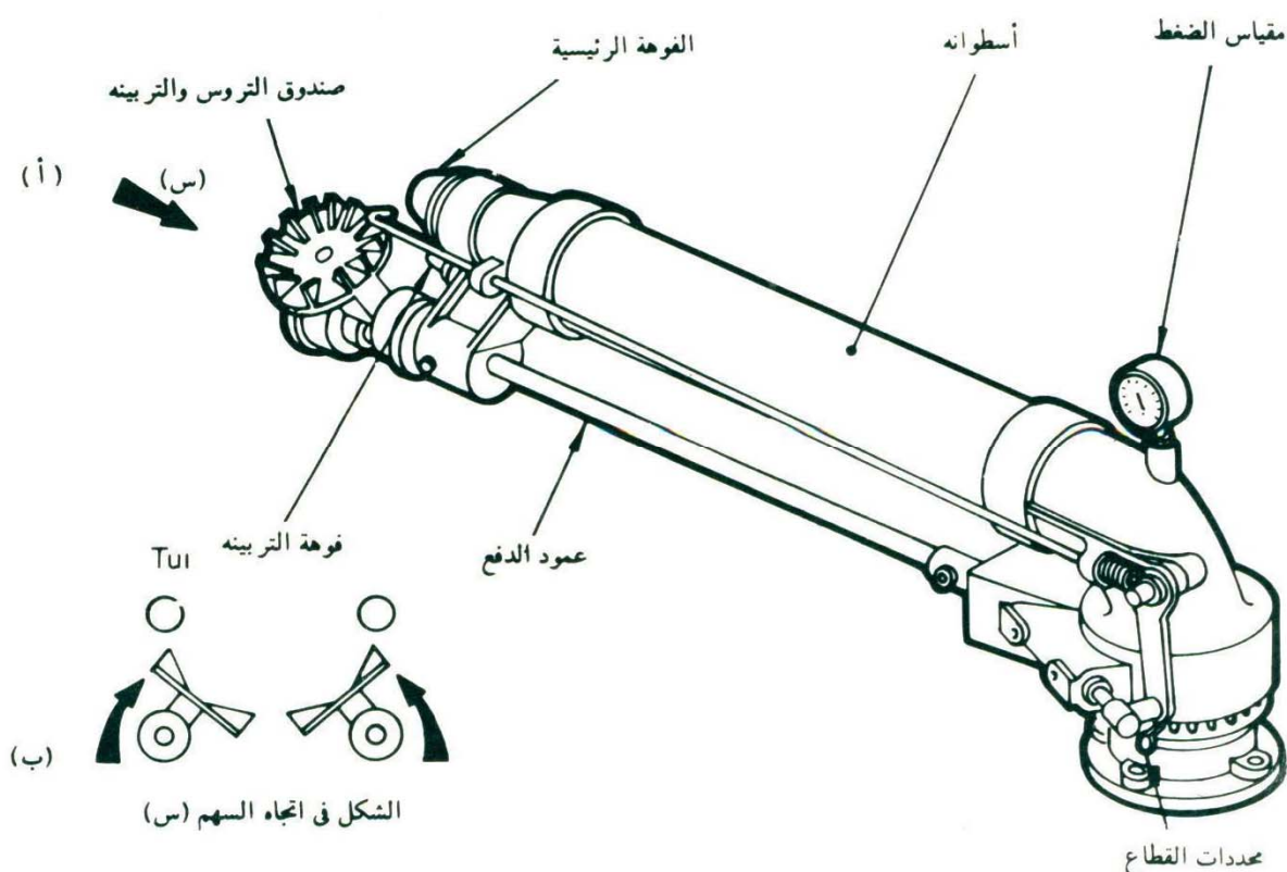
شكل (٣ - ٤) مدفع الرش ذو التربين المائي
