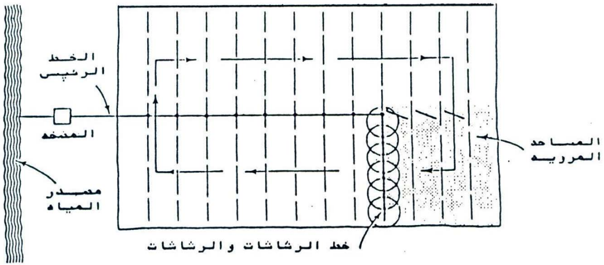
١. نظام متنقل يحرك يدويا وبه خط رشاشات واحد
