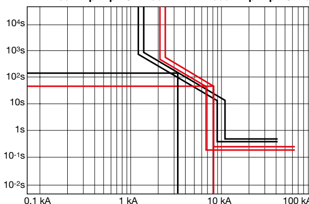
E1.2B 1250 Ekip Dip LSI 1250 - E2.2N 2500 Ekip Dip LSI 2500
