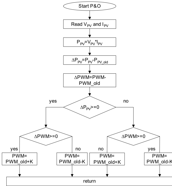
Fig. 6. P&amp;O MPPT algorithm.
