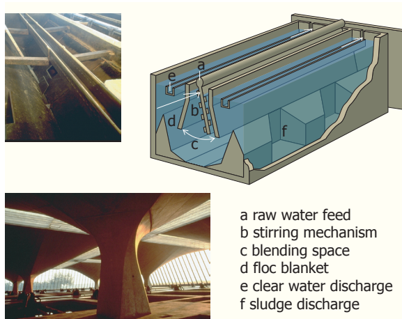
Figure 28 - Floc blanket installation at Berenplaat
