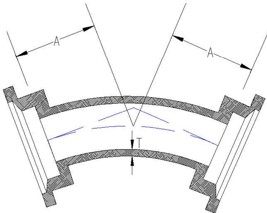
45° BENDS
