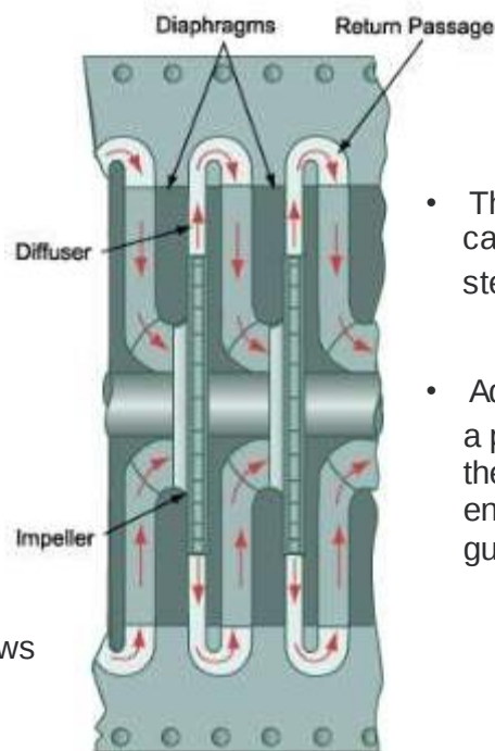
Diaphragms
