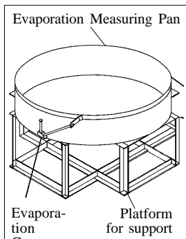
U.S. PAN-A. - Evaporimeter
