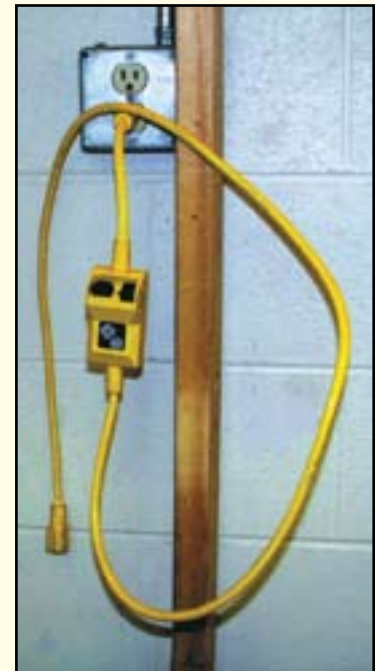
Portable GFCI.
