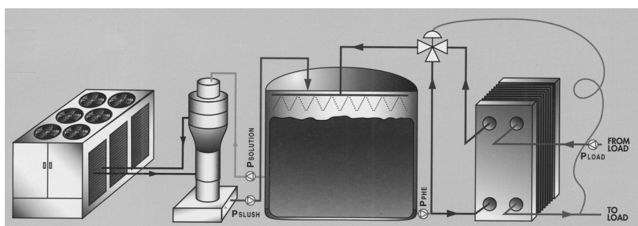
Figure 9. Typical ice slurry configuration. (d)
