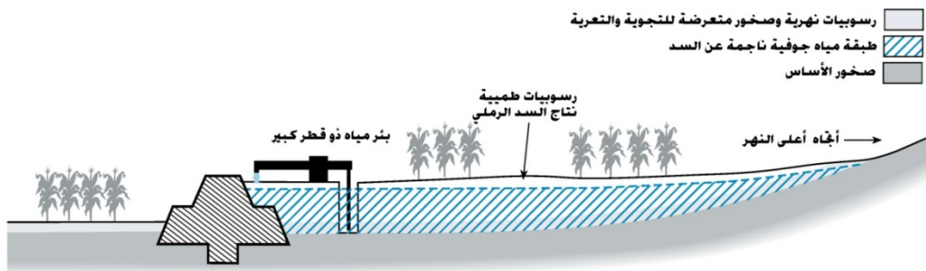
الشكل (10.5) قطاع طولي للسد الرملي (From Foster and Tuinhof, 2004)
