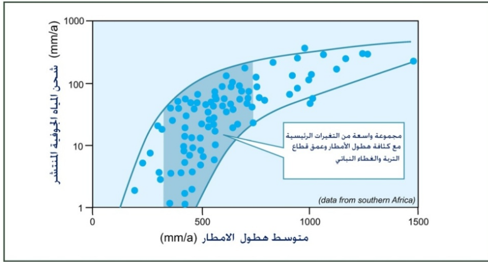
شكل (2.4) تقدير معدل الشحن (التغذية) مقابل هطول الأمطار السنوي (GW•MATE, 2002-2006)
