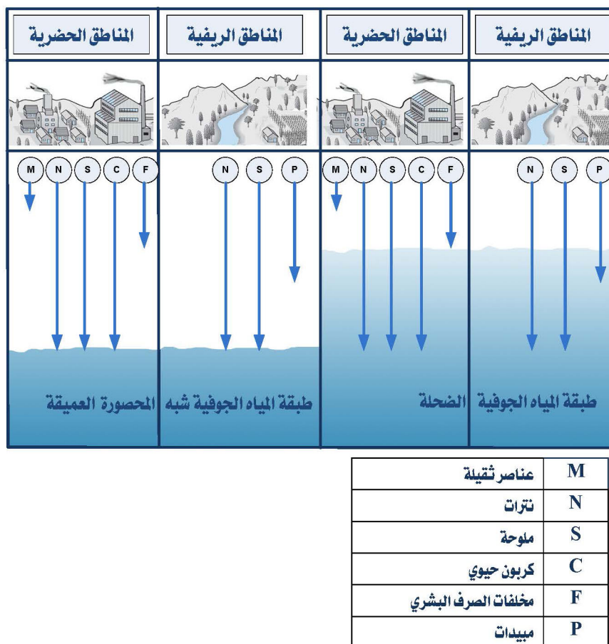
الشكل (8.2) مخاطر المياه الجوفية هي مزيج من مخاطر التلوث وقابلية المياه الجوفية للتلوث (تحويل من الناشر) و (GW•MATE,2002-2006)
