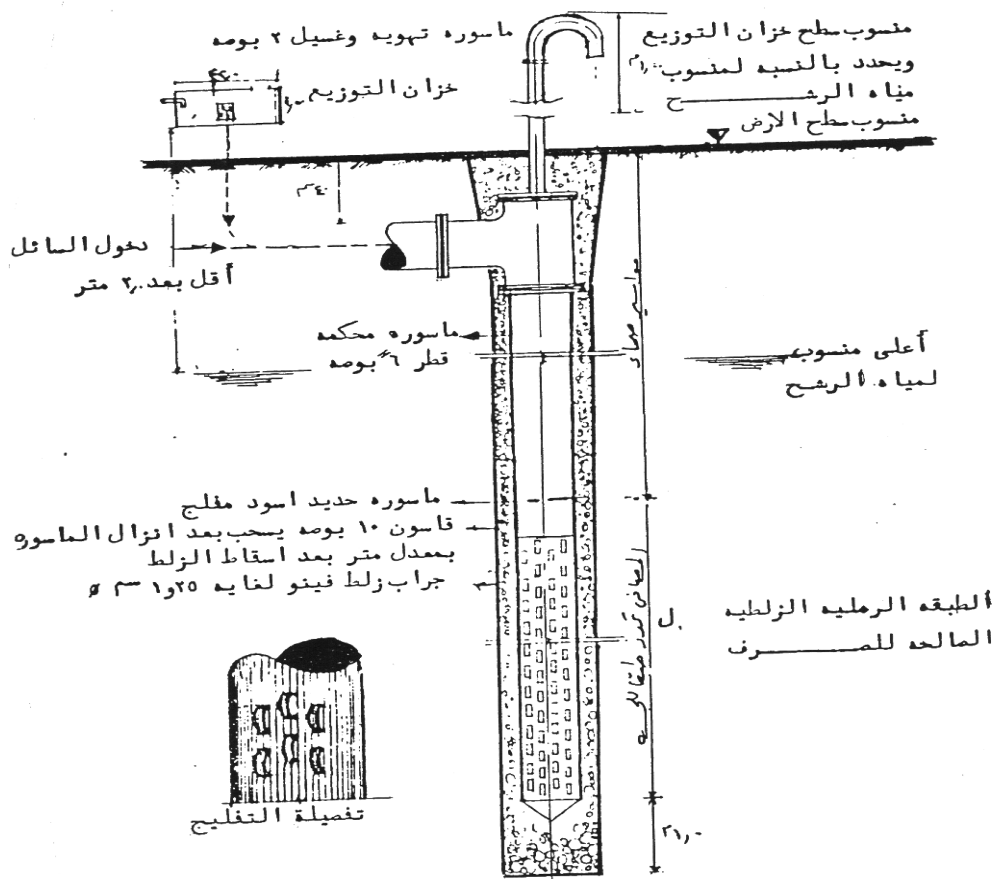
شكل رقم (7) تفاصيل آبار التصريف العميقة - قيسون الصرف
