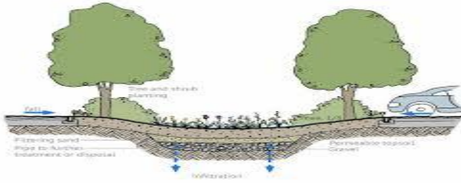
شكل رقم (8) تفاصيل خندق الترشيح الرملي
