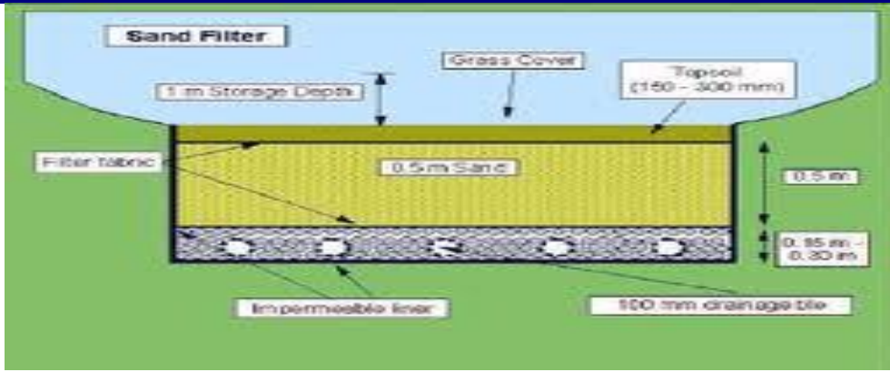
شكل رقم (9) تفاصيل الخنادق الرملية تحت سطح الأرض
