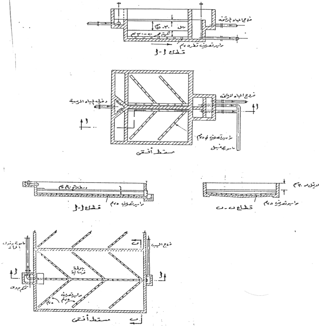
شكل رقم (12) تفاصيل المرشحات بطيئة الانسياب
