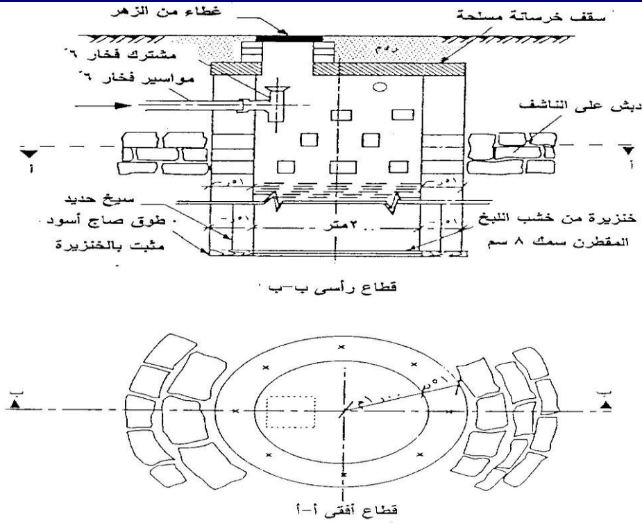
شكل (5) تفاصيل بئارة التصريف في باطن الأرض للتخلص من السيب
