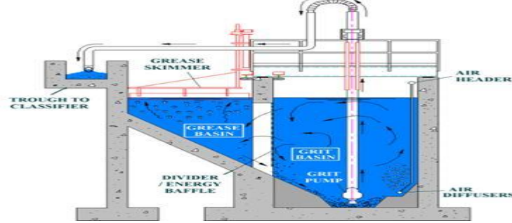
شكل رقم (13) تفاصيل غرف حجز الزيوت والشحوم والرمال
