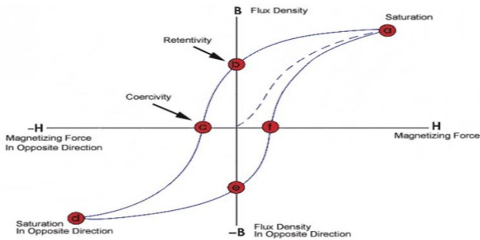
شكل رقم (٤) يوضح منحنى التخلف المغناطيسي
