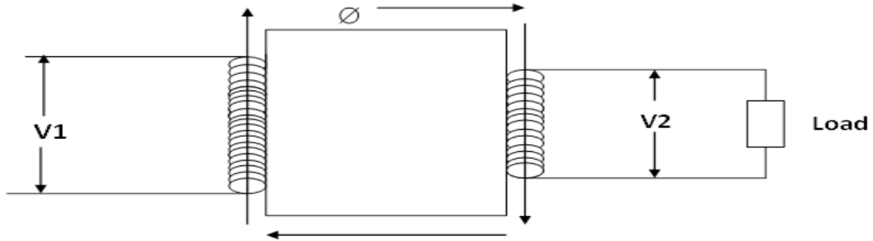
شكل رقم (١) يوضح محول أحادي الوجه
