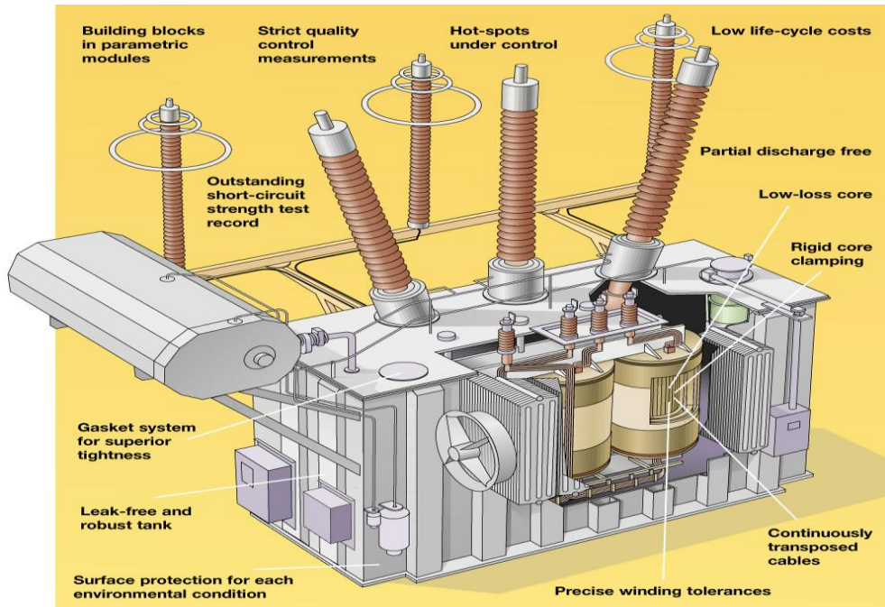
شكل رقم (٢) يوضح تركيب محول القدرة الكهربائي
