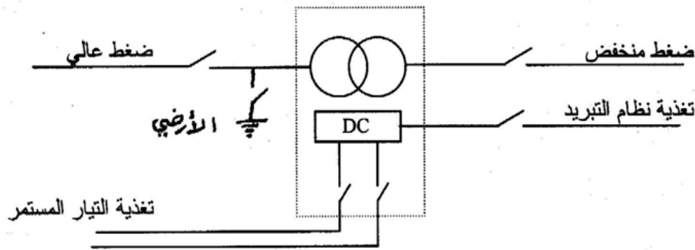
تغذية نظام التبريد بالتيار المستمر
