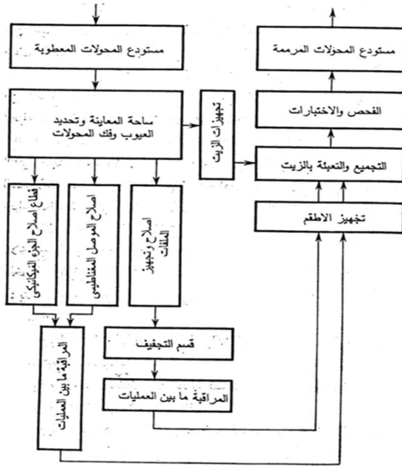
مخطط إصلاح محول تبريد زيتي
