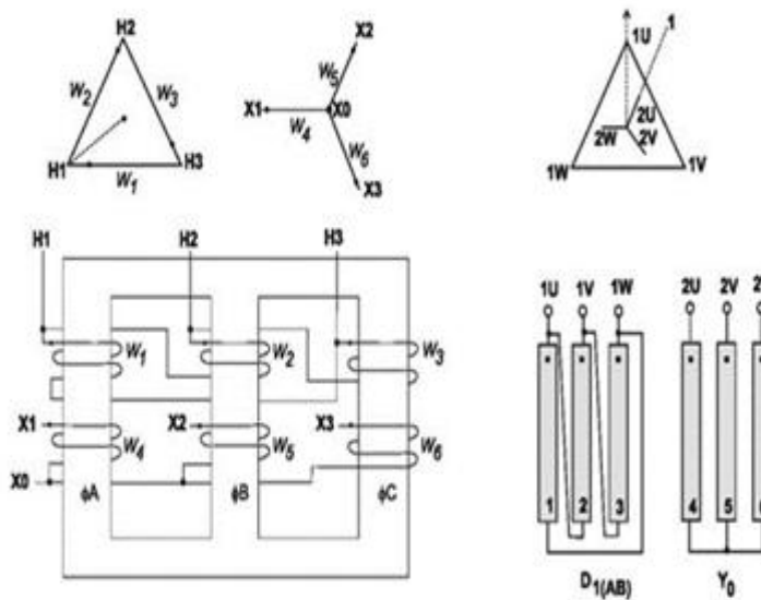
Dy1 ( D_{1(AB)} - Y_0 )
