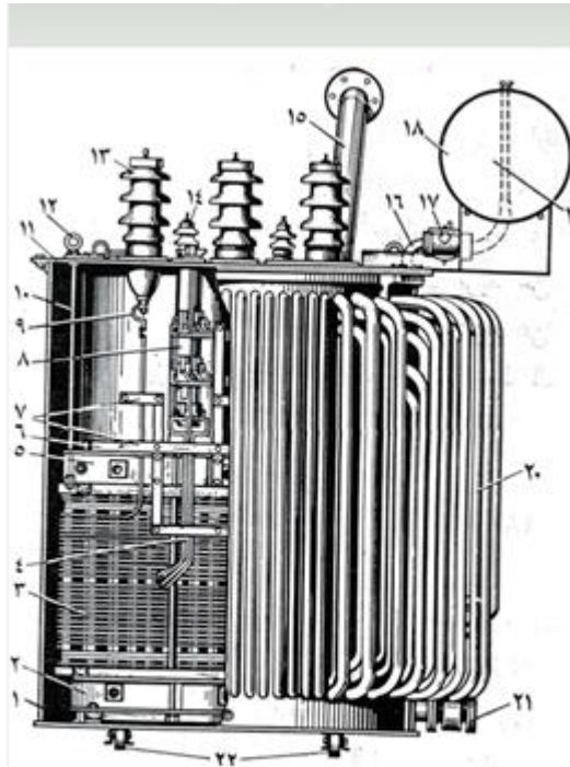
شكل رقم (17) يوضح محول ثلاثي الاطوار، ثلاثي الملفات من الحجم الثالث نو تبريد زيتي
