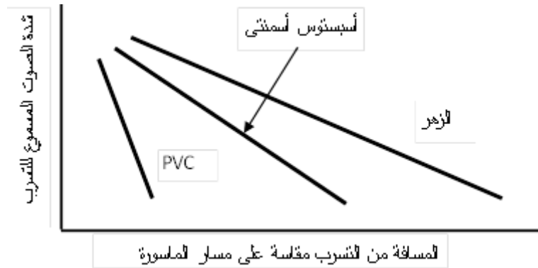
شكل رقم (١) العلاقة بين شدة اصوات التسرب المسموعة خلال جدار الماسورة ونوعية مادة الماسورة
