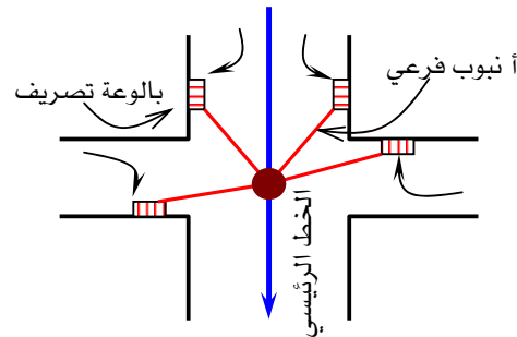
الشكل (٧,٣): تصريف مياه الأمطار في تقاطع طريق
