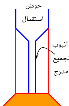
شكل (٧- ١): جهاز قياس المطر
