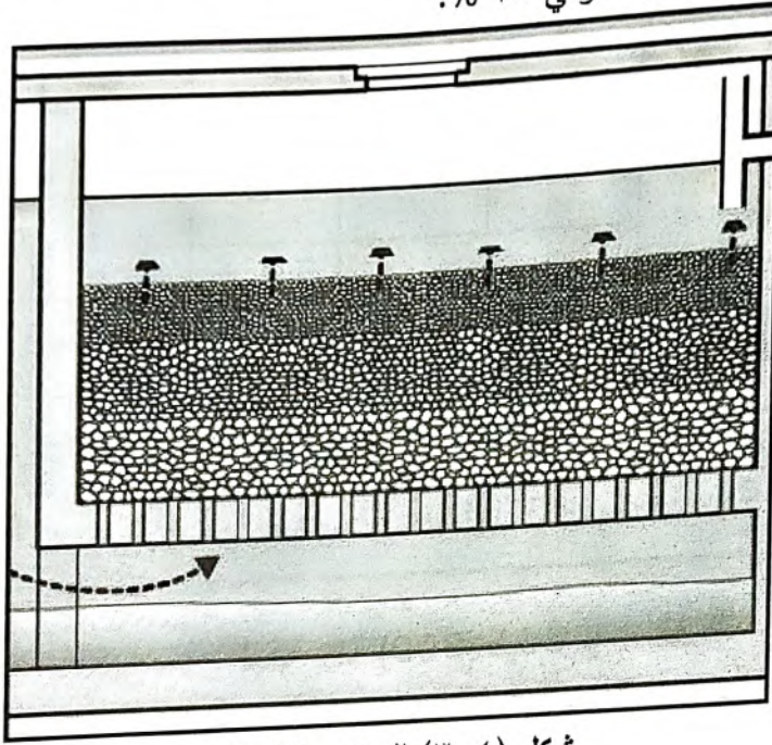
شكل (٤-٣) المرشح اللاهوائي
