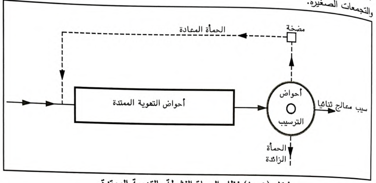
شكل (٥-١) نظام الحمأة النشطة بالتهوية الممتدة
