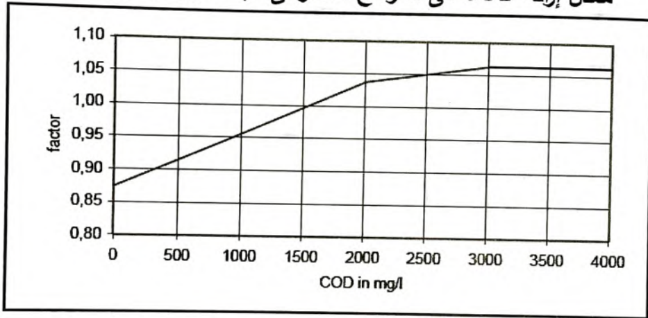
نسبة إزالة COD داخل المرشح اللاهوائى طبقاً لقيمة COD فى مياه الصرف الخام
