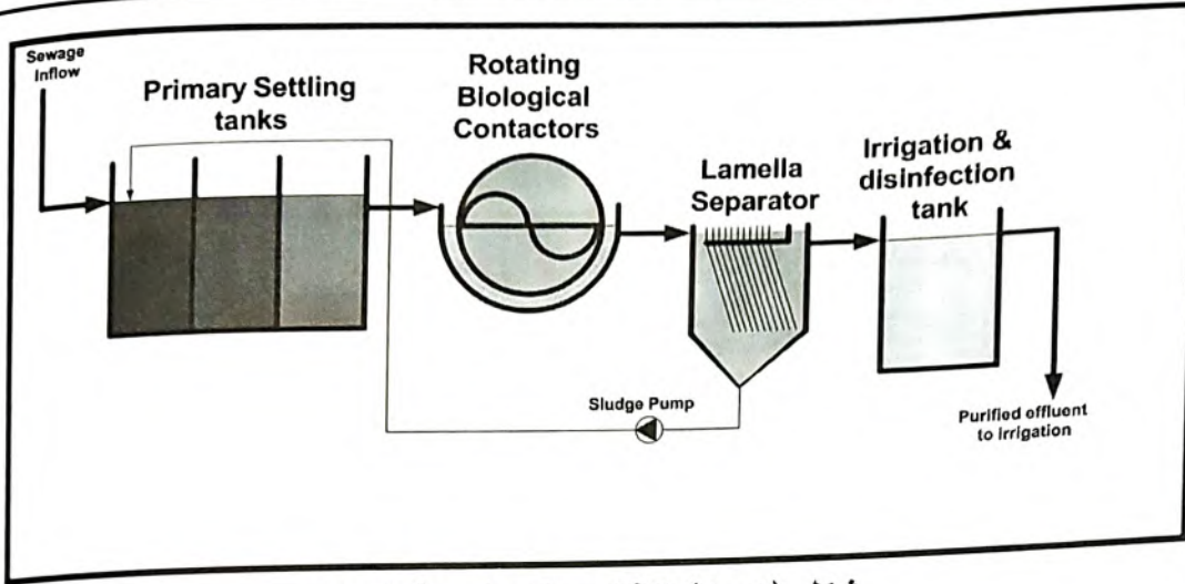
شكل (٥-٤) الأقراص البيولوجية الدوارة
