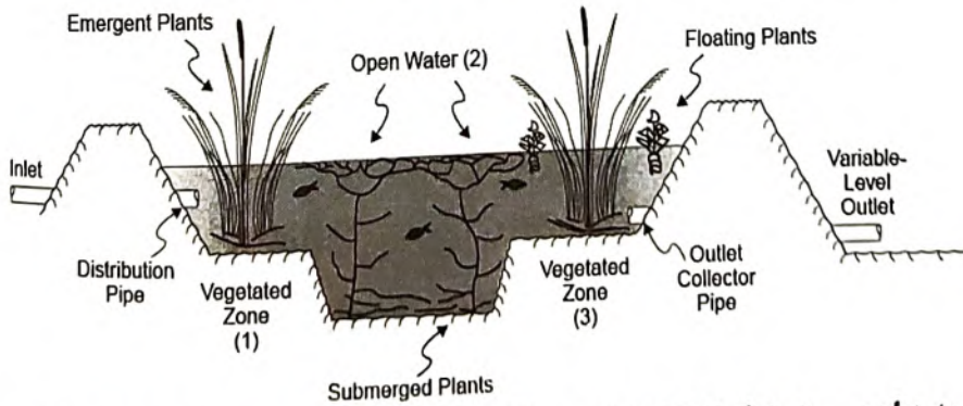
شكل (٨-٥) الأراضي الرطبة (FWS) المدمجة ذات غطاء خضري مع مناطق مفتوحة لسريان المياه
