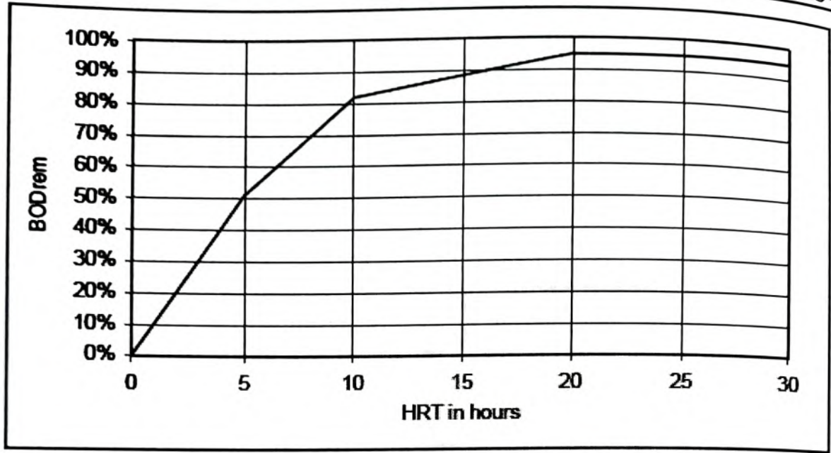
نسبة إزالة (BOD) طبقا لزمان المكث
