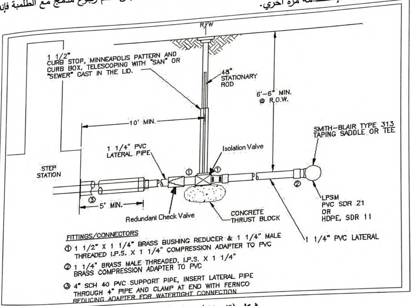
شكل (٢١-٣) منظومة التوصيل
