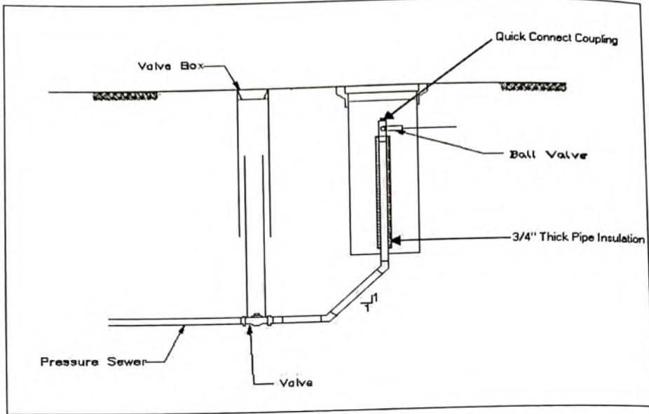
شكل (٣-٢٠) وصلات الغسيل
