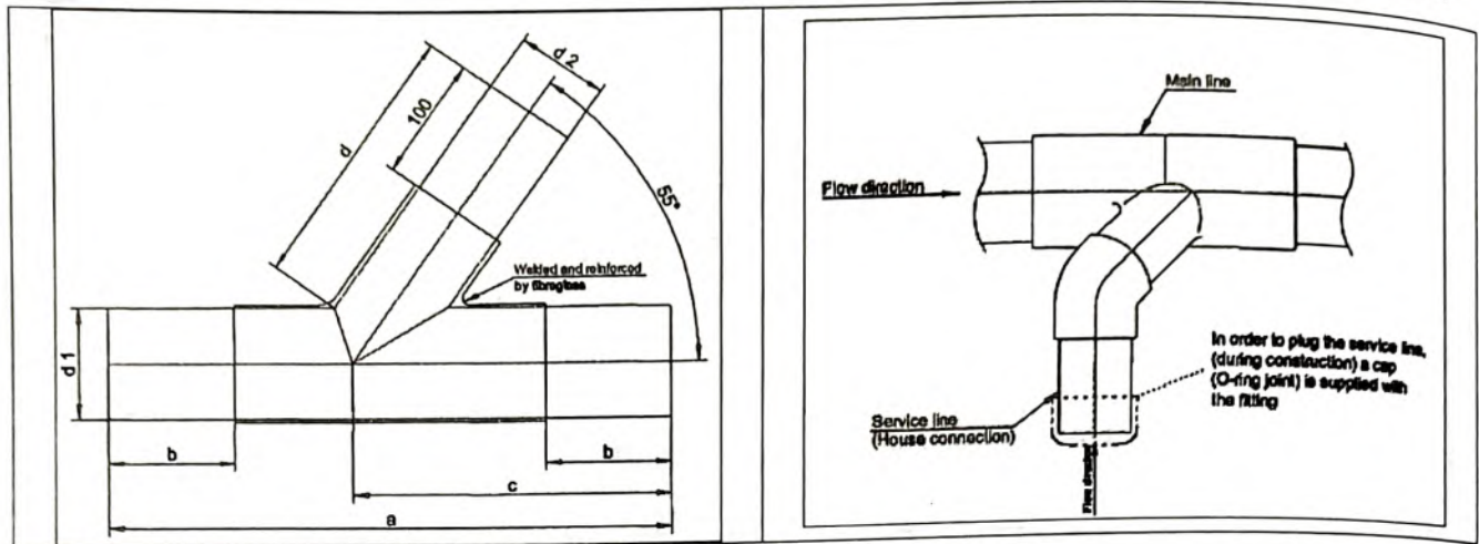
شكل (٣-١٦) قطعة خاصة للوصلات ٥٥٥
