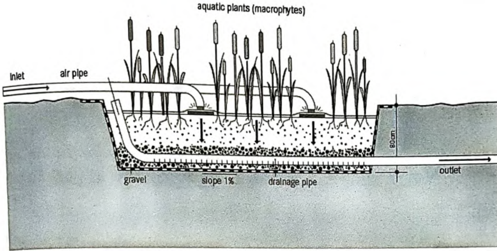
شكل (٥-١٠) الأراضي الرطبة بطريقة التدفق تحت السطحي الرأسية
