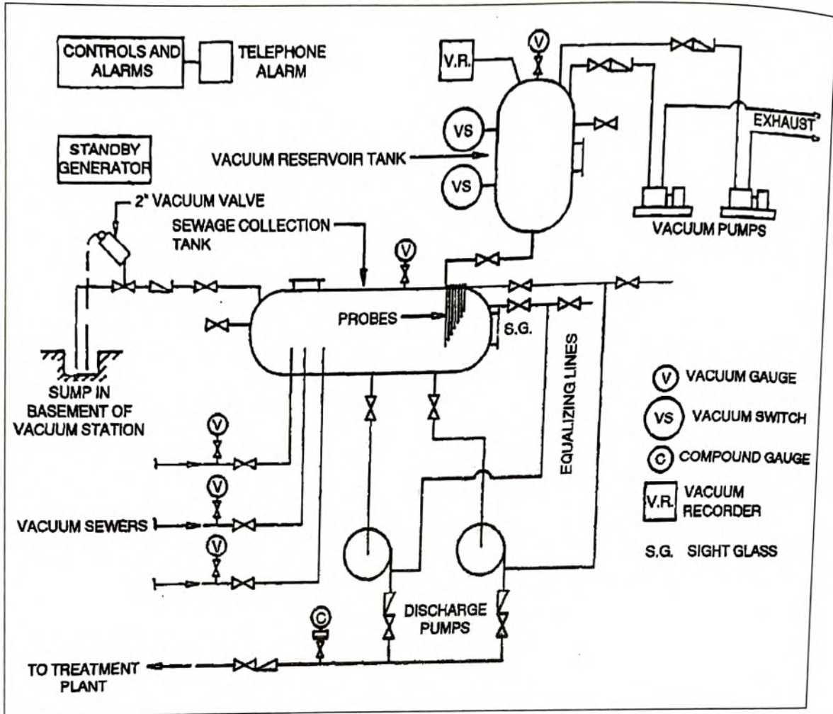
شكل (٣-١١) مكونات محطة توليد ضغط التفريغ
