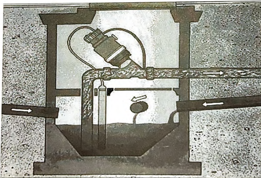
شكل ( ٣-٩ ) مثال لمحبس التفريغ
