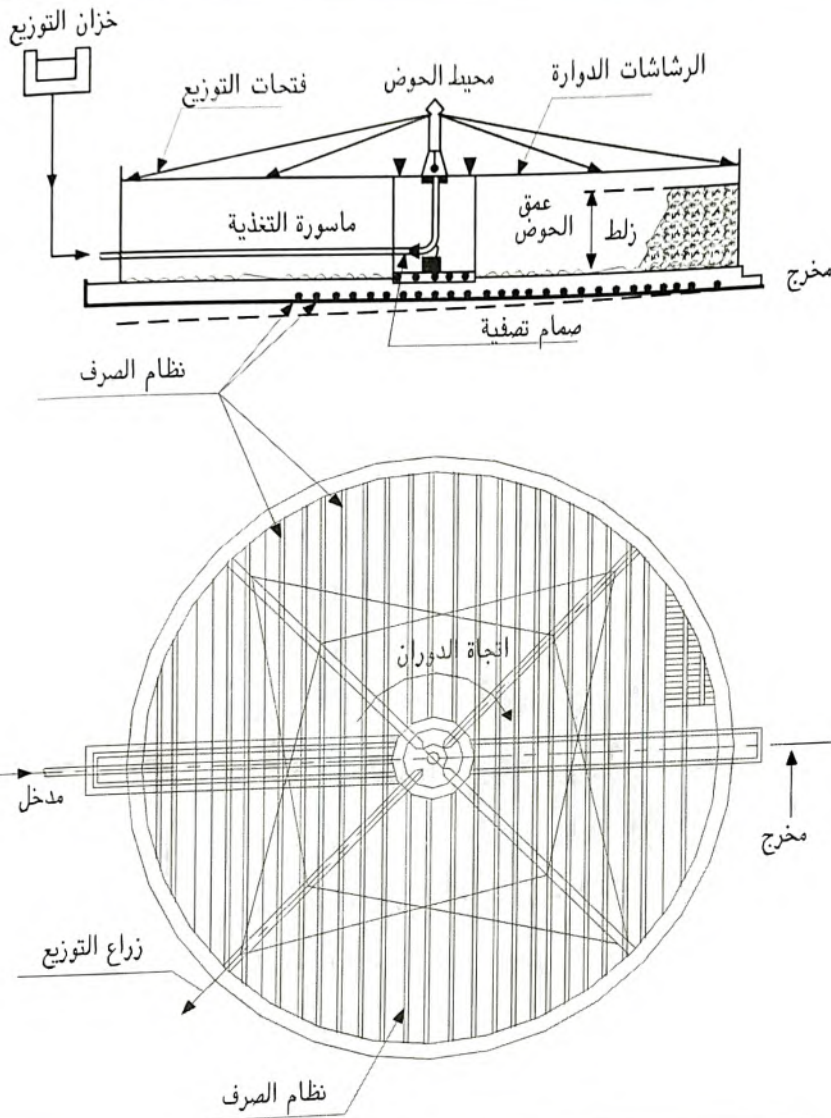
شكل (٥-٣) المرشحات الرملية
