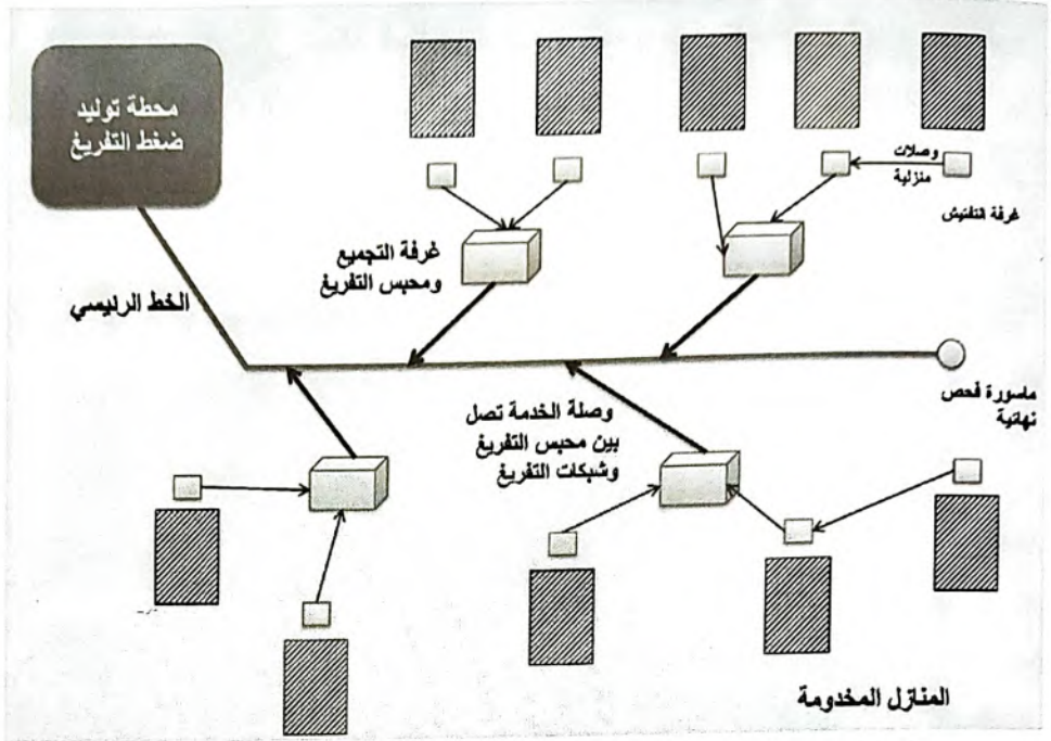
شكل ( ٣-٨ ) مكونات نظام شبكات الصرف الصحي بتفريغ الهواء
