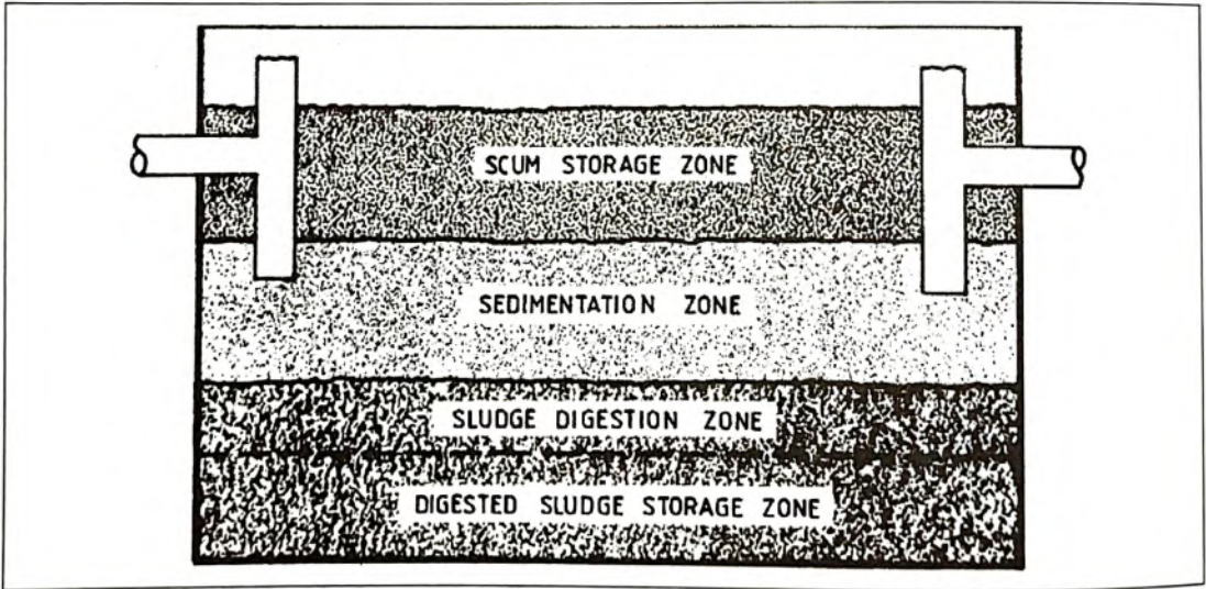
شكل (١-٤) المناطق المختلفة داخل خزان التحليل
