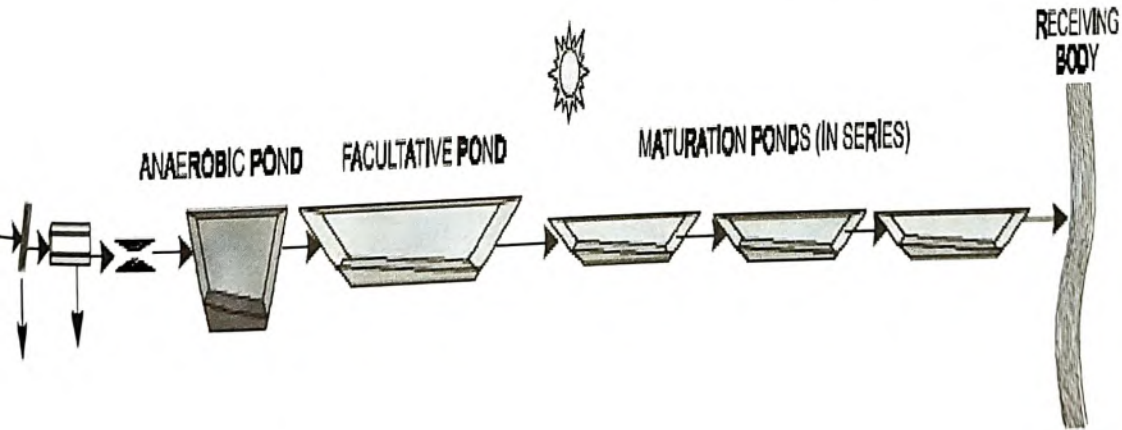
شكل (٦-٥) مراحل برك الأكسدة الطبيعية
