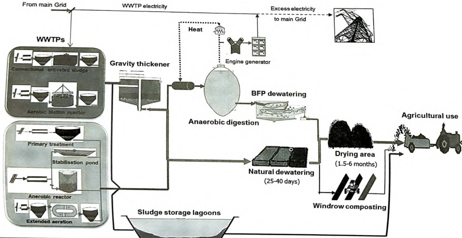
شكل (٦-٢) مخطط لمراحل وترتيب أعمال معالجة الحمأة
