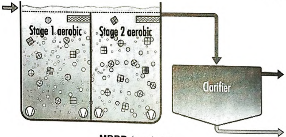
شكل (٥-٥) MBBR
