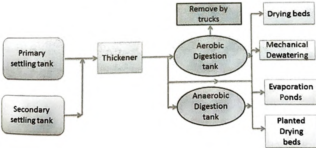
شكل (١-٦) مخطط لعمليات معالجة الحمأة
