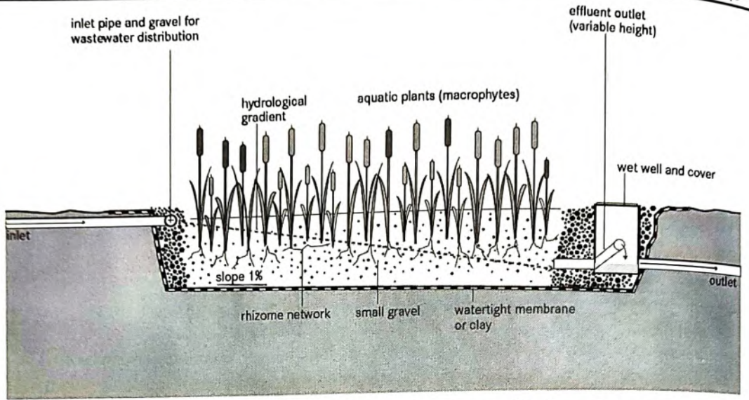
شكل (٥-٩) الأراضي الرطبة بطريقة التدفق تحت السطحى الأفقية
