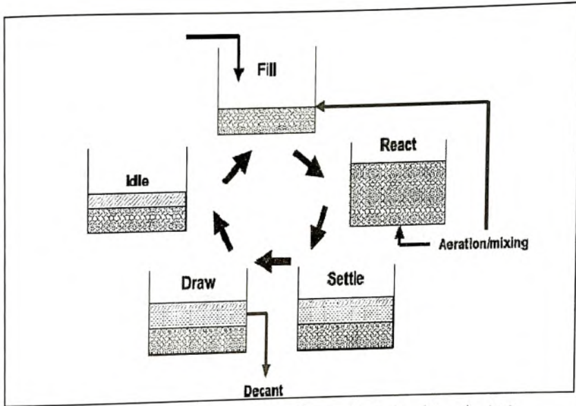
شكل (٢-٥) مراحل المعالجة باستخدام نظام الدفعات المتتالية
