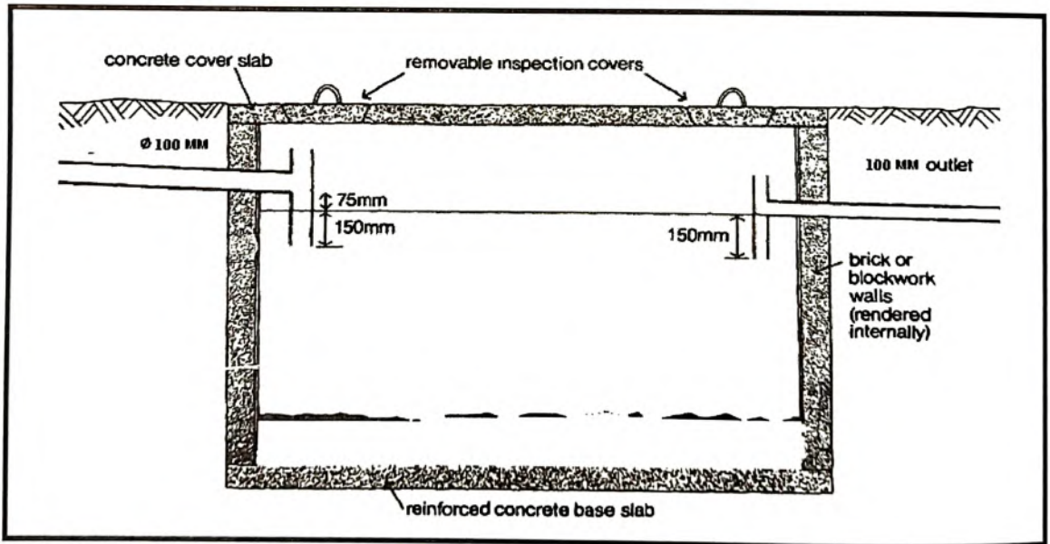
شكل (٣-٧) مثال لخزان استقبال من الخرسانة المسلحة
