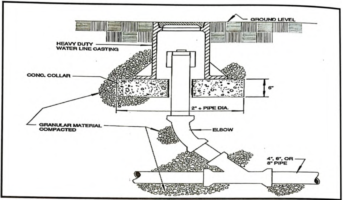
شكل (٣-٣) مقطع رأسي لتركيب طبقة التسليك
