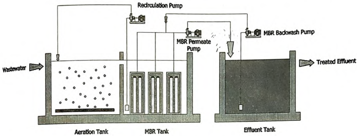
شكل (١١-٥) نموذج لوحدة مدمجة تعمل بنظام الأغشية
