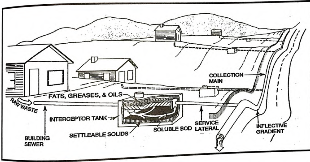
شكل (١-٣) عناصر ومكونات نظام الصرف الصحى ذو الاقطار الصغيره
