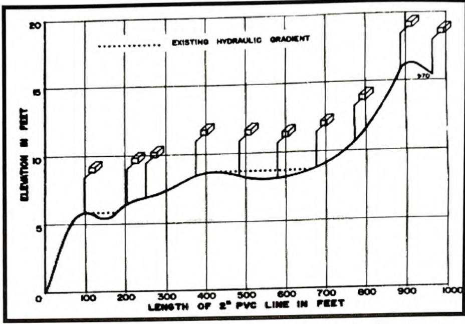
شكل (٣-٢) مثال على الميل الهيدروليكي لمسورة بنظام الأقطار الصغيرة
