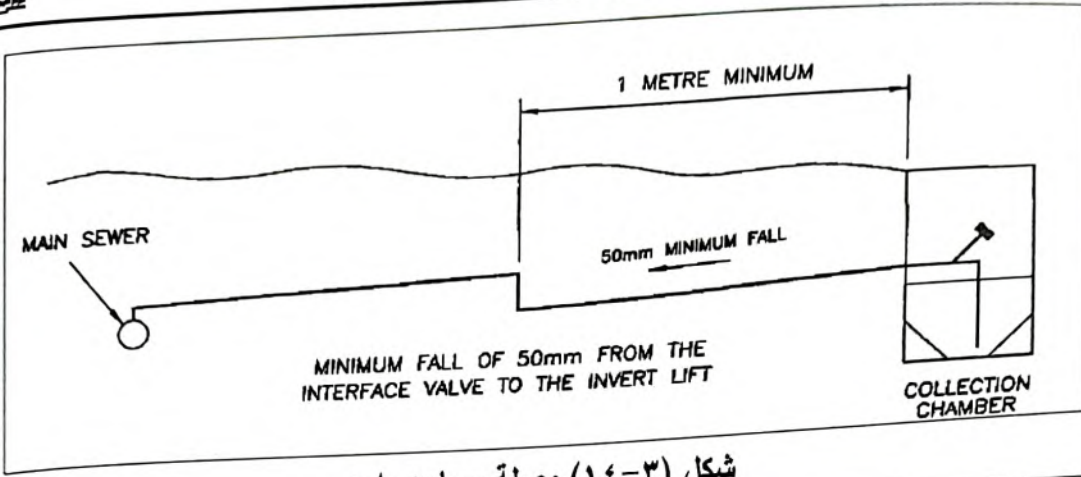
شكل (٣-١٤) وصلة بصاعد واحد
