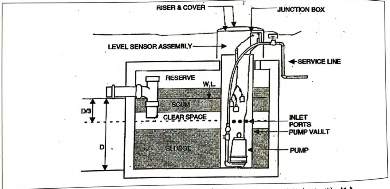
شكل (٣-٢٢) التقسيم المختلف لمنطقة تجمع الزيوت والشحوم ومنطقة تجمع الحمأة
