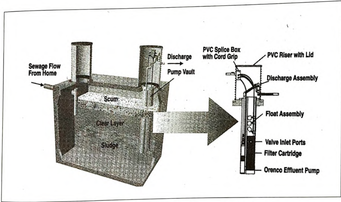
شكل (٣-١٧) نموذج لخزان التحليل مع نظام STEP
