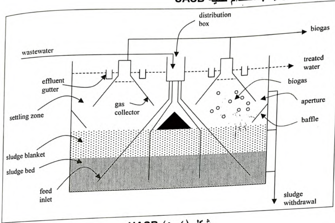
شكل (٤-٥) UASB
