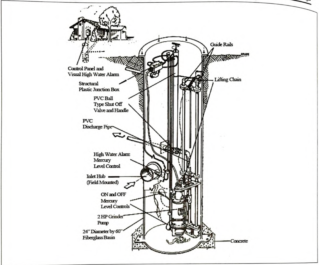
شكل (٣-١٨) نموذج للمطبق بنظام GP
