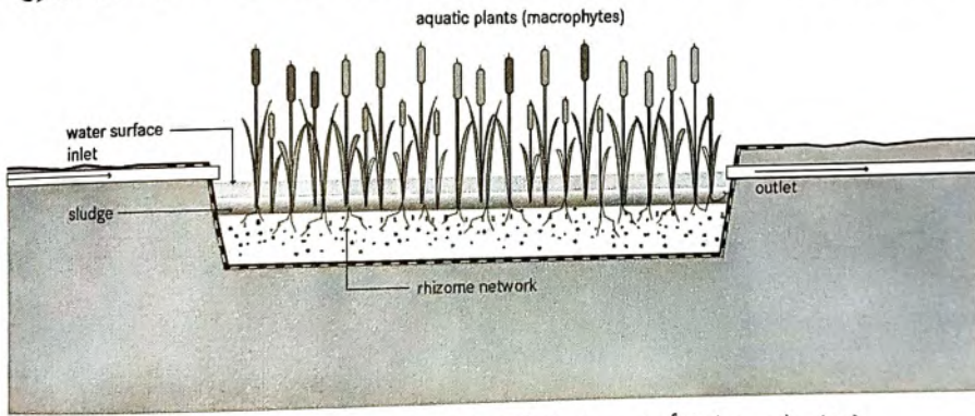
شكل (٧-٥) الأراضي الرطبة (FWS) ذات غطاء خضري فقط
