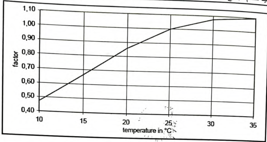
معدل إزالة COD فى المرشح اللاهوائى طبقاً لدرجة الحرارة
