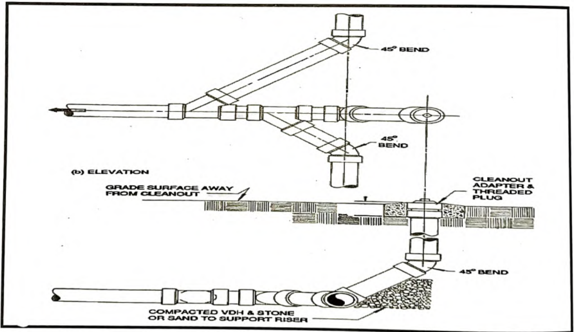
شكل (٣-٤) مقطع أفقي ومقطع رأسي لاتصال طبقة التسليك على عدة خطوط
