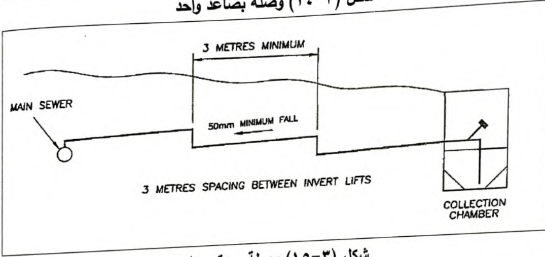
شكل (٣-١٥) وصلة بعدة صواعد
