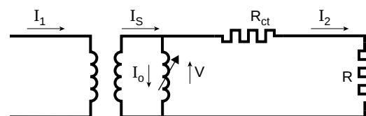
Fig. 9 : CT equivalent diagram.
