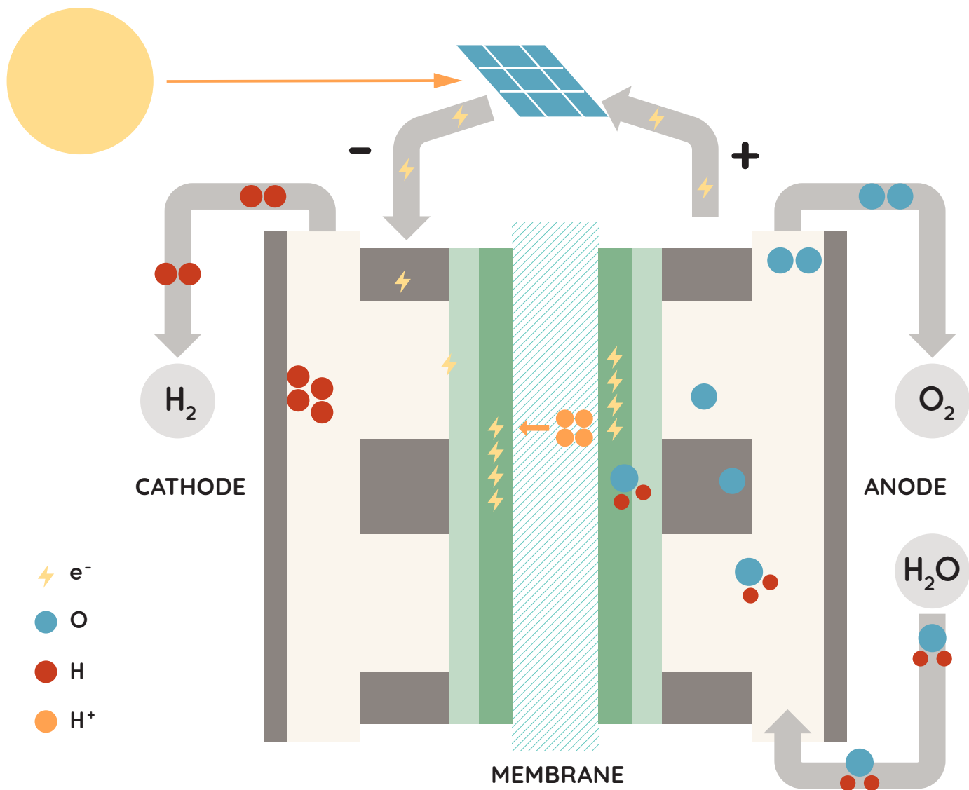
PEM electrolyser [25].
