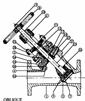
OBLIQUE
