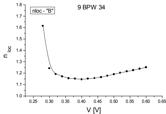
Fig. 5. Method "B" (Vasic et al, 2005).
