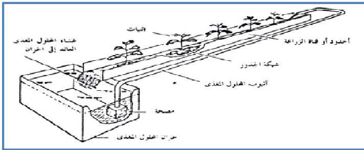
صورة (٣٣): توضيح التصور العام لكيفية تصميم قناة الزراعة في تقنية الغشاء وحركة المحلول المغذي على شكل غشاء رقيق فيها
