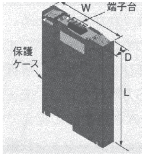
Fig. 19. EDLC case unit-160 V, 3.7 F, 50 A, 8.8 kg, W: 272 mm, L: 387 mm, D: 51 mm
