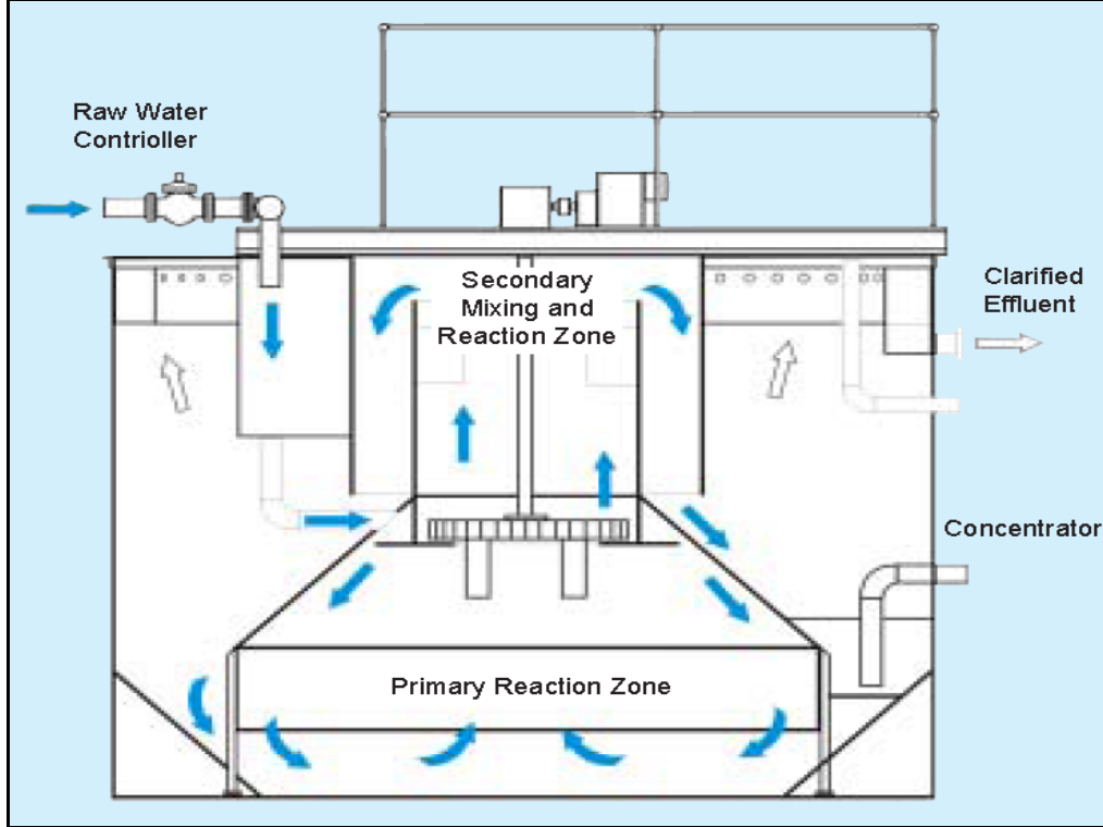
شكل (٢١-٢) أحواض الترويب والترسيب السريعة (Accelerator)
