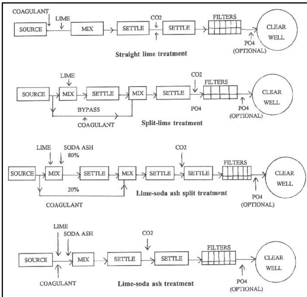
شكل (٢-٣٩) أساليب إزالة العسر من المياه
