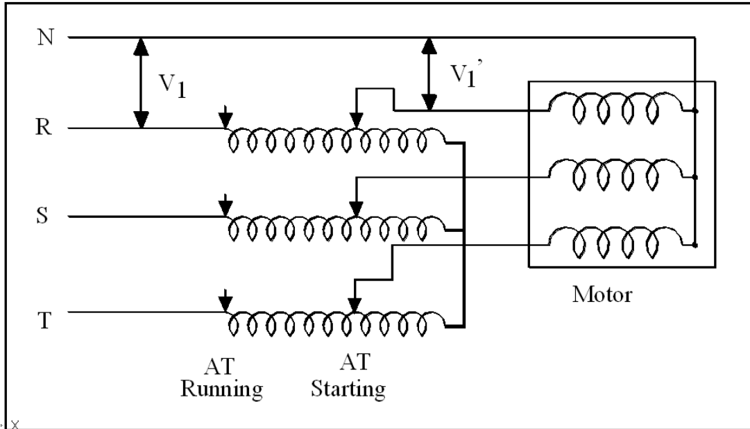
شكل (٤-٣) البدء باستخدام محول أوتو
