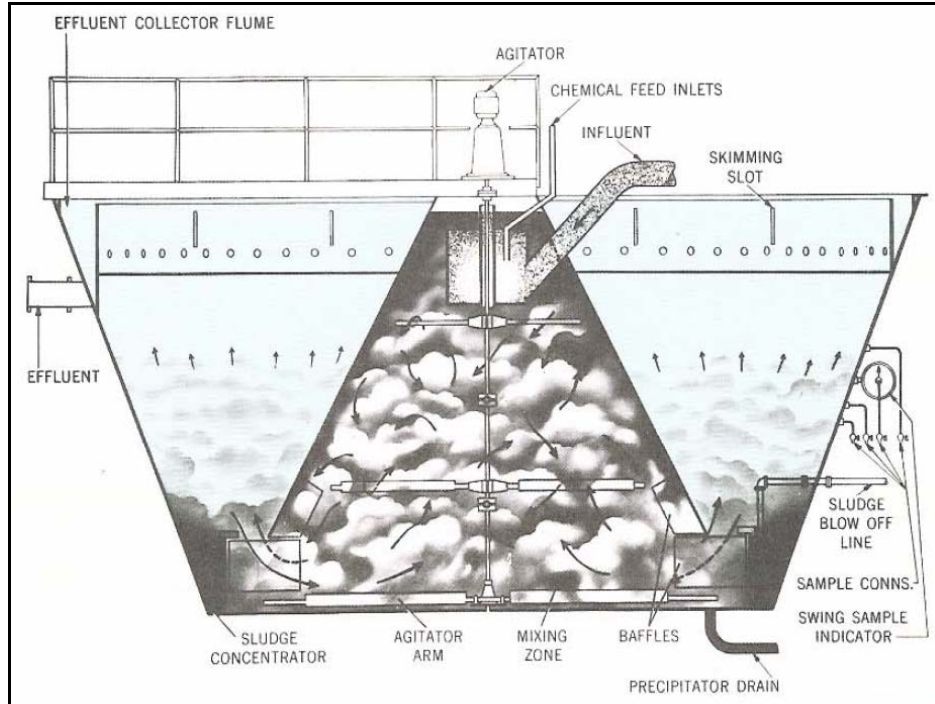
شكل (٢٢-٢) أحواض الترويق والترسيب السريعة (Preceptor)
