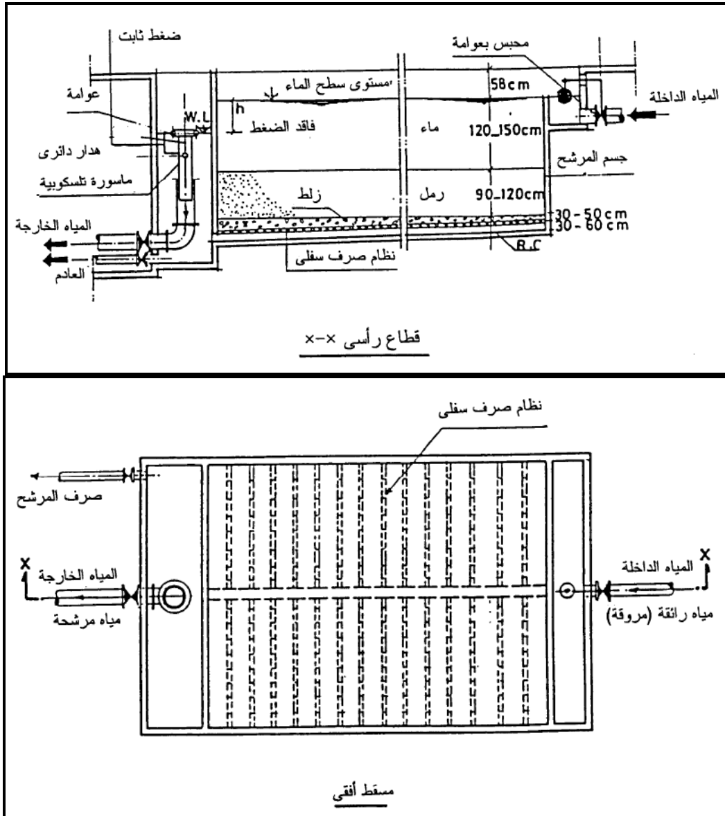
شكل (٢-٢٦) المرشحات الرملية البطيئة
