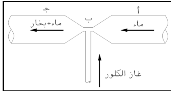
شكل (٢-٣٥) الحاقن
