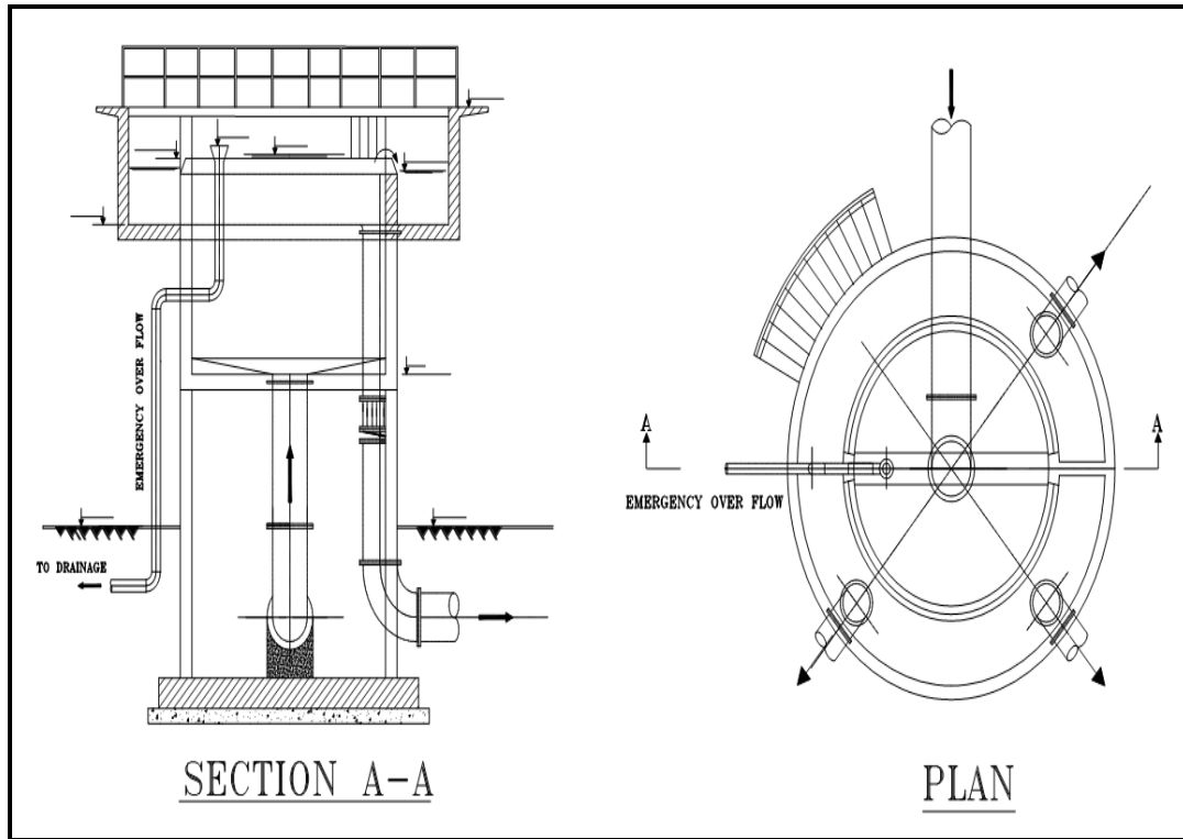
شكل (٢-٩) بئر التوزيع
