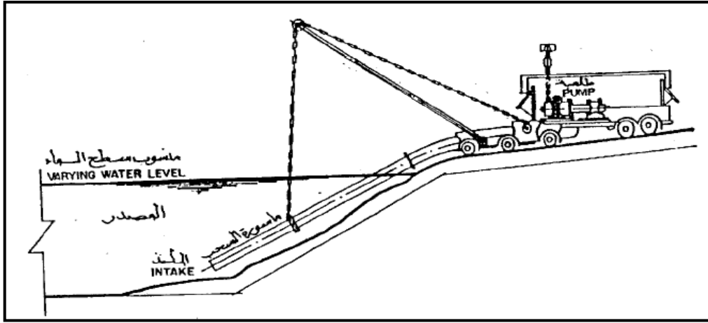
شكل (٦-٢) المآخذ المؤقت
