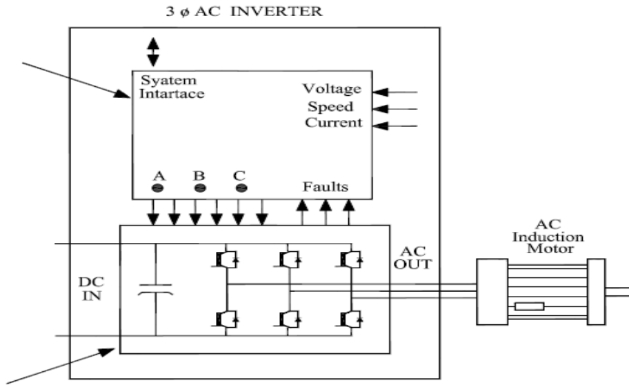
شكل (٧-٤) قالبية جهد ثلاثية الطور
