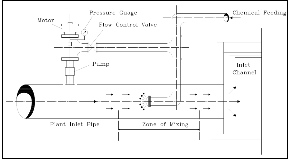
شكل (١٢-٢) مضخة تغذية فى خط مواسير المياه الرئيسى
