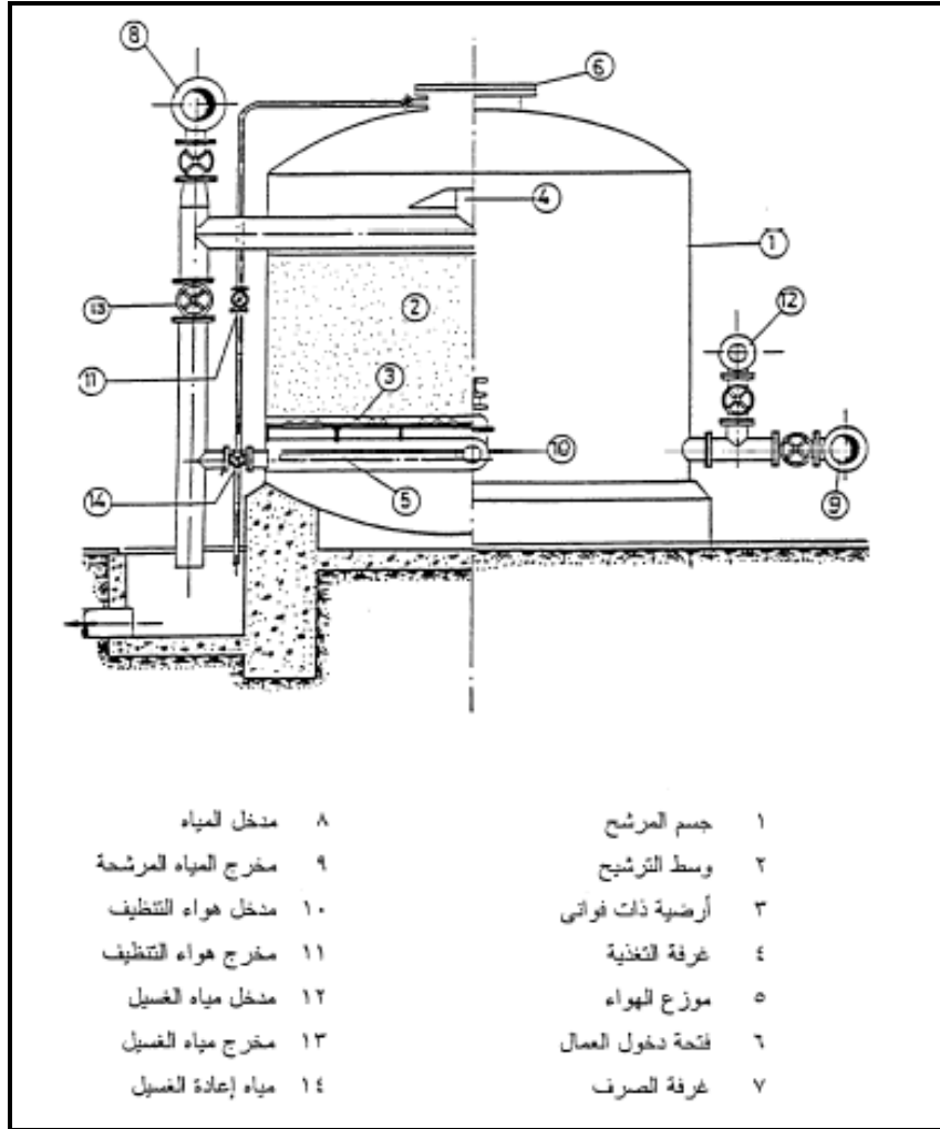
شكل (٢-٣٣) تفاصيل مرشح ضغط رأسى
