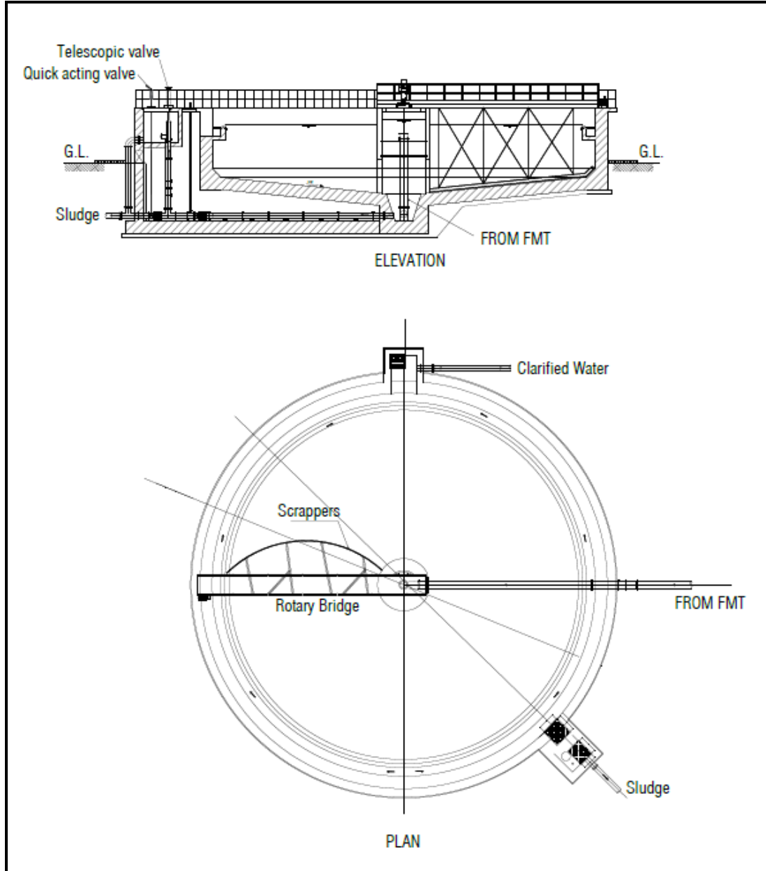
شكل (١٩-٢) حوض الترسيب الدائرية
