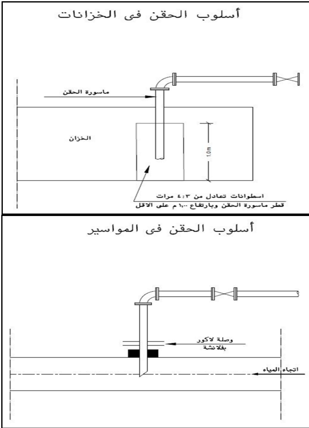
شكل (٢-٣٦) الحقن فى المواسير أو الخزانات
