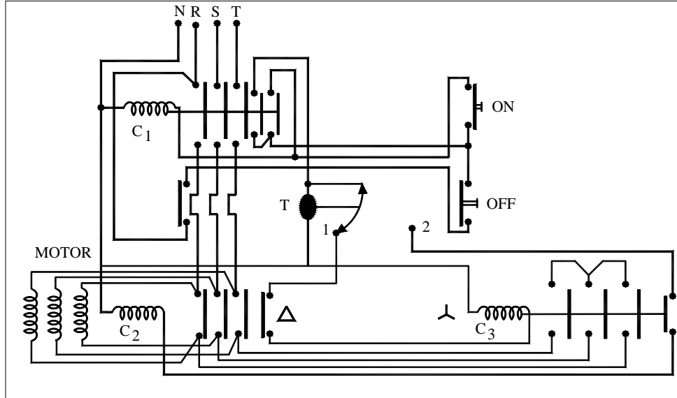
شكل (٤-٥) نظام اتوماتيكي نجمة دلتا باستخدام الكنتاكتور
