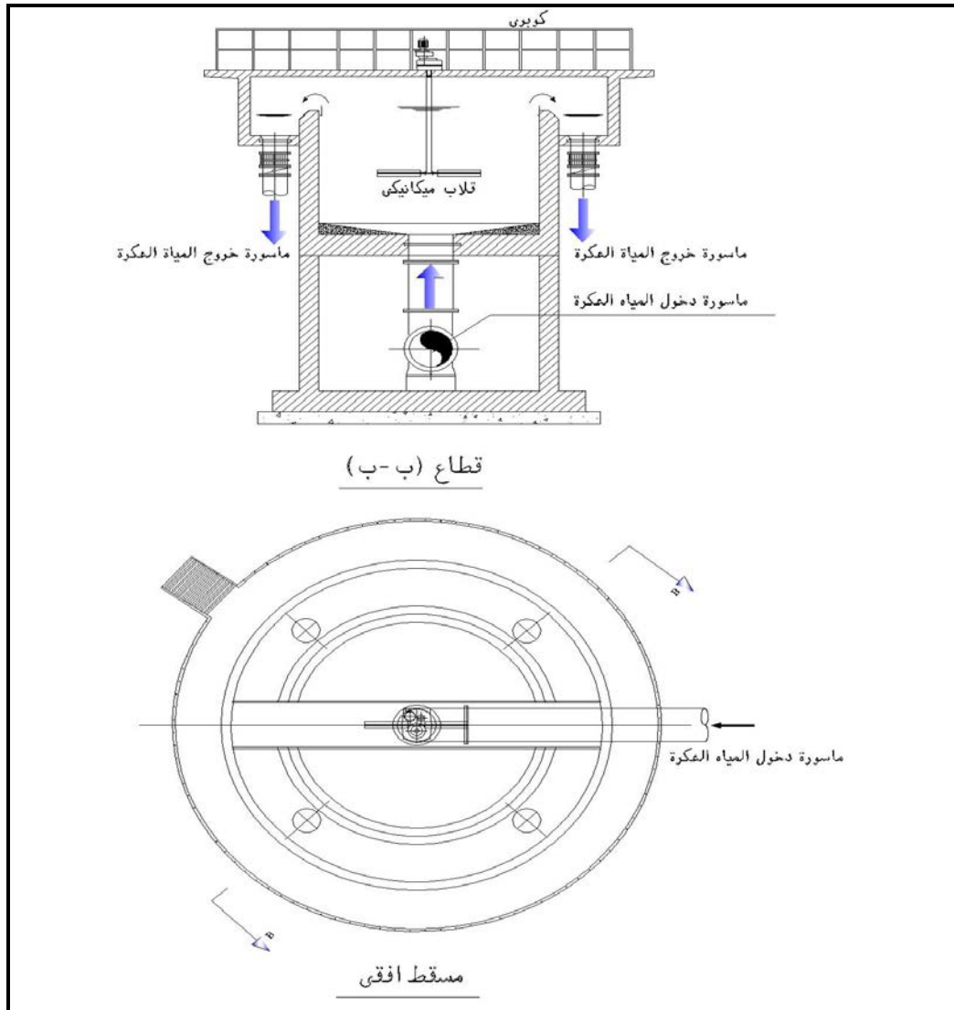
شكل (٢-١٠) حوض الخلط السريع
