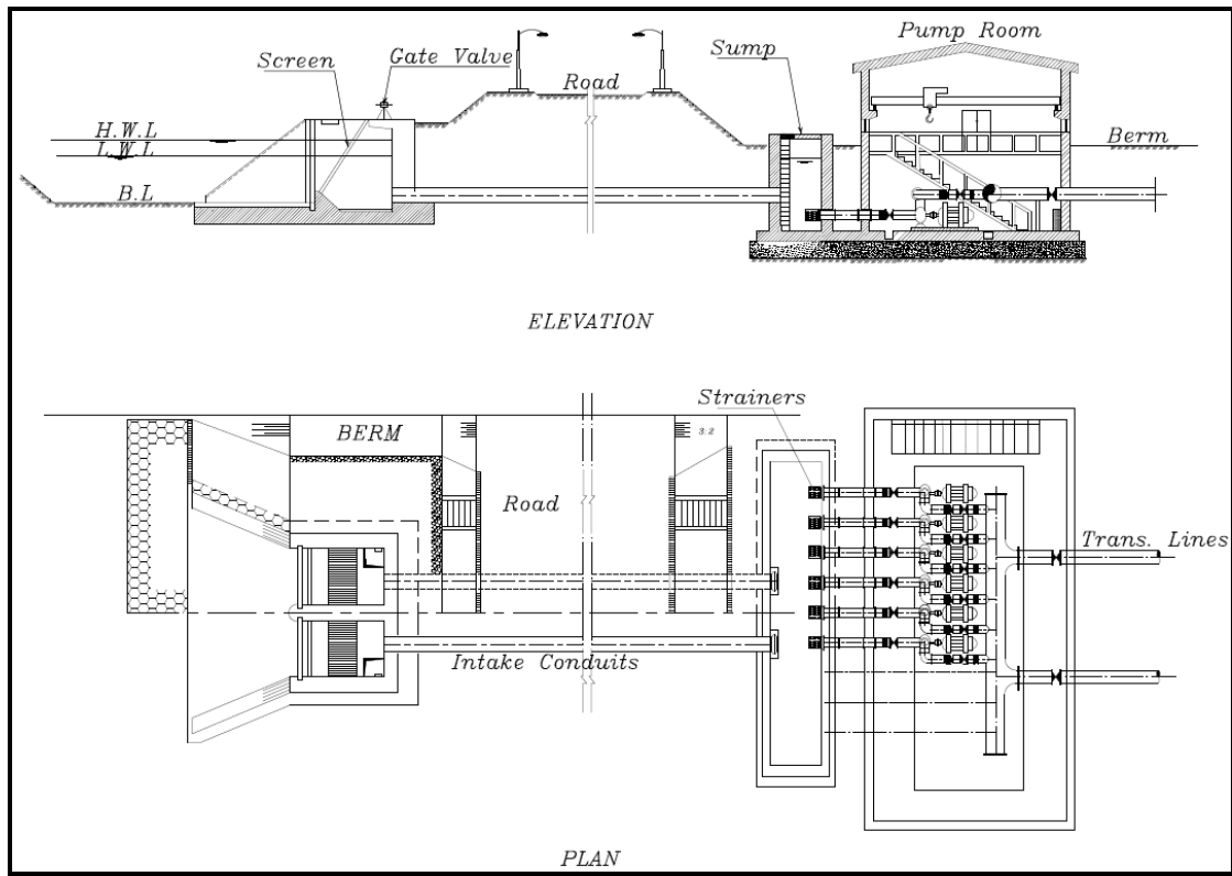
شكل (٢-٢) مأخذ الشاطئ
