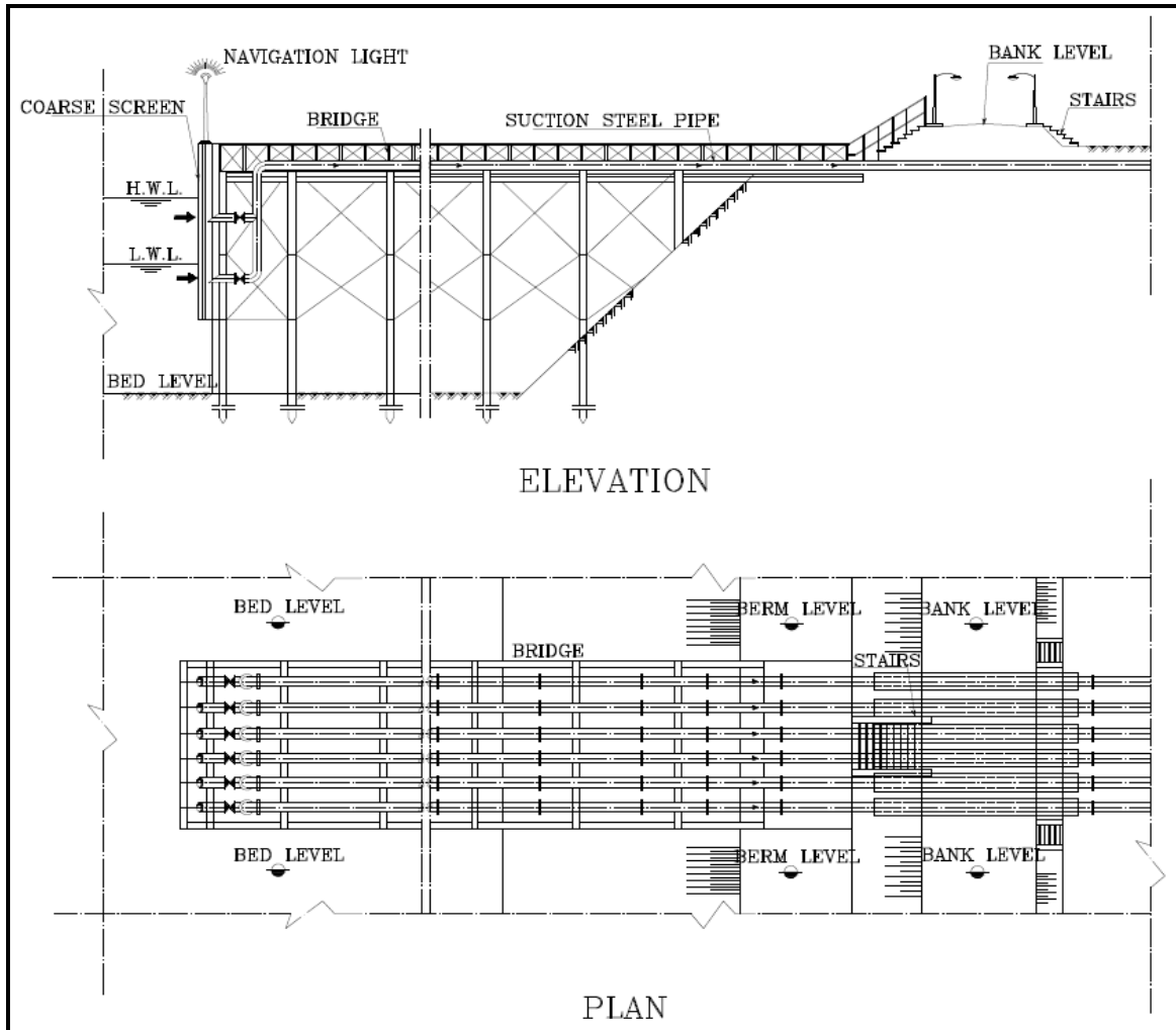
شكل (١-٢) مأخذ الماسورة
