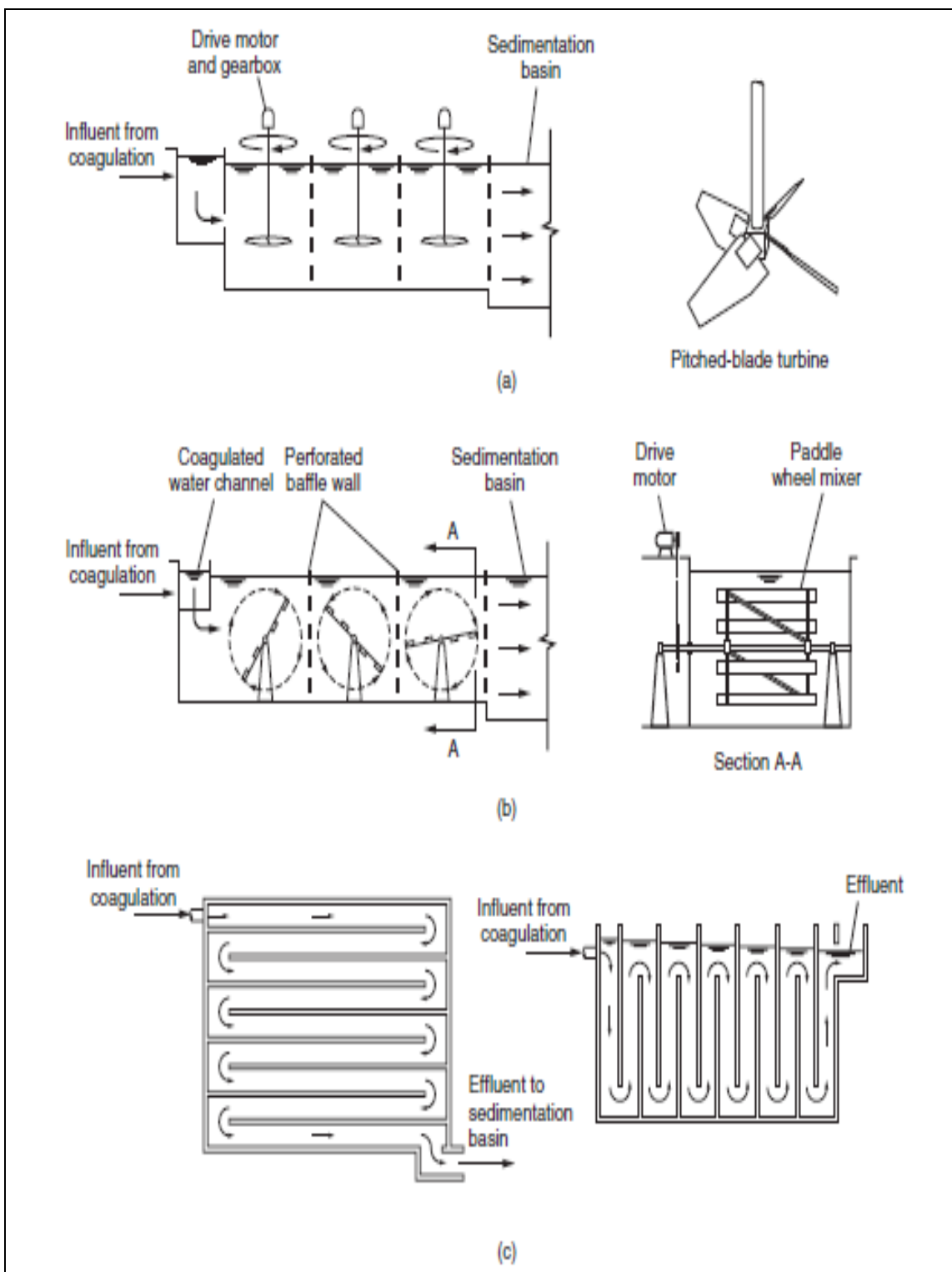
شكل (٢-١٥) أنواع القلابات الميكانيكية المستخدمة فى الخلط البطئ
