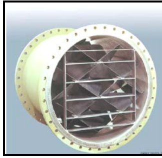
شكل (١٣-٢) الخلط الإستاتيكي بالمواسير
