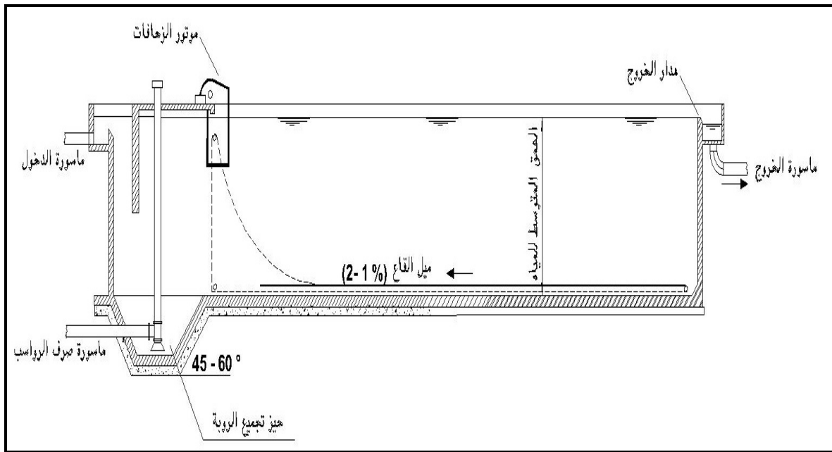
شكل (٢-١٦) حوض الترسيب المستطيل
