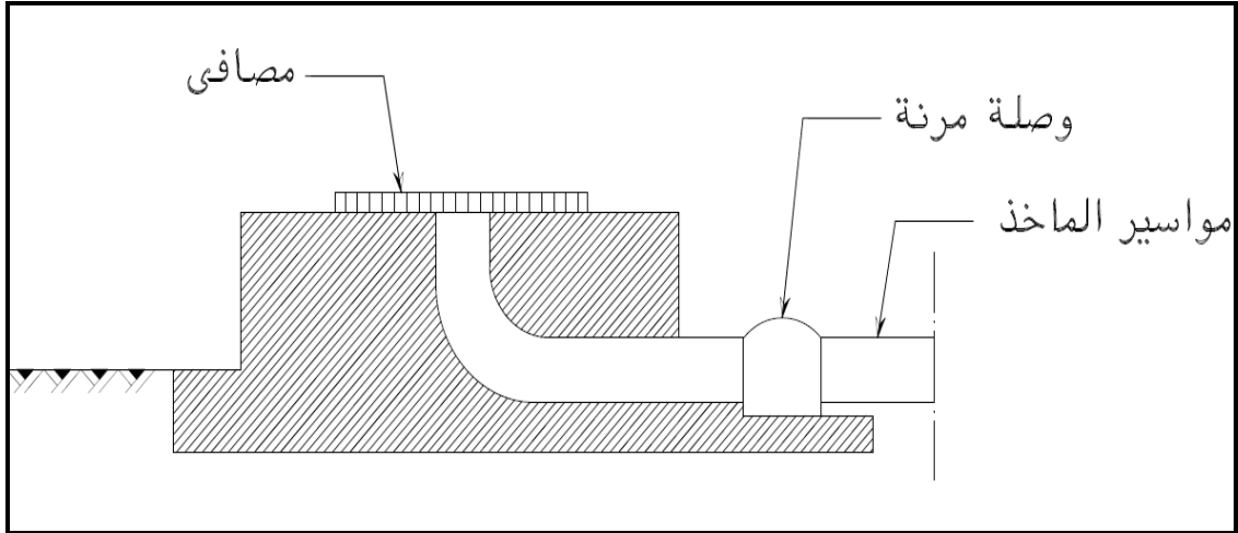
شكل (٢-٤) المآخذ المغمور (النموذج الثانى)
