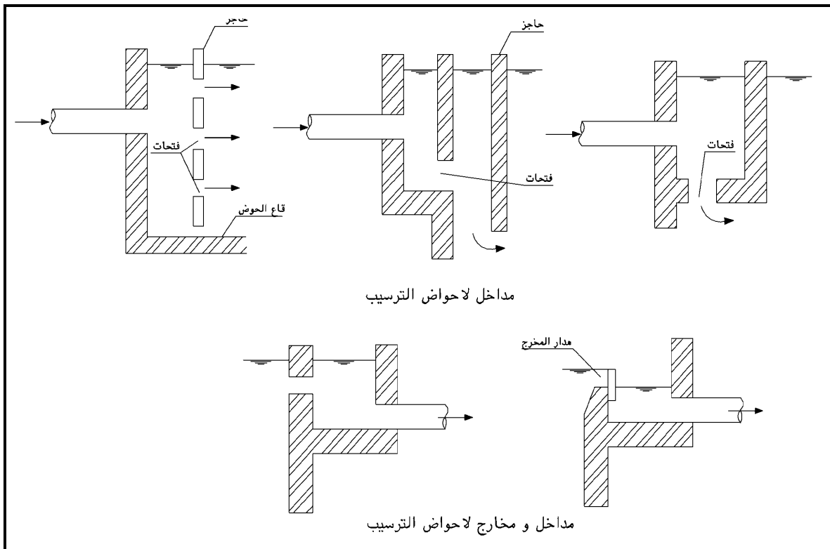
شكل (٢-١٧) مداخل ومخارج لأحواض الترسيب
