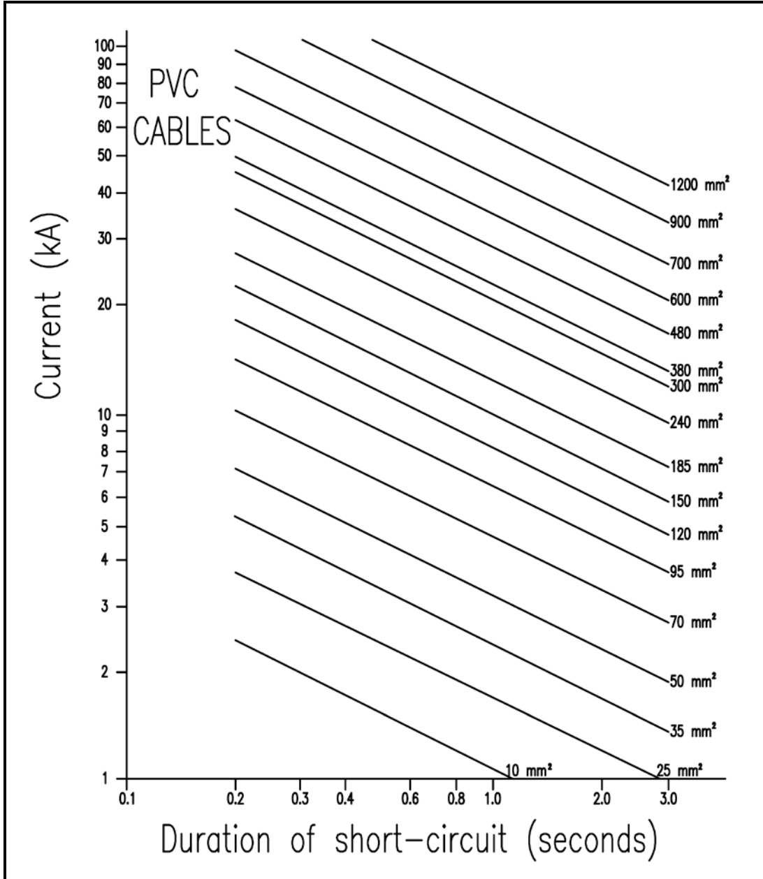
شكل (٤-١٥) نوموجرام العلاقة بين تيار القصر والزمن ومساحة المقطع للموصلات المستخدمة فى حالة الكابلات المعزولة بمادة PVC (للكابلات ذات الموصلات النحاسية ضغط منخفض).
