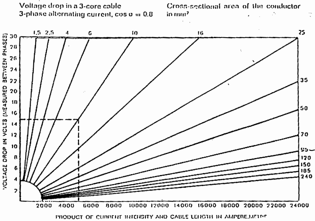
شكل (٤-١٣) نوموجرام حساب التنزيل في الجهد للكابلات ثلاثية الأقطاب لإمرار التيار المتردد ثلاثي الوجه عند معامل قدرة واحد صحيح.
