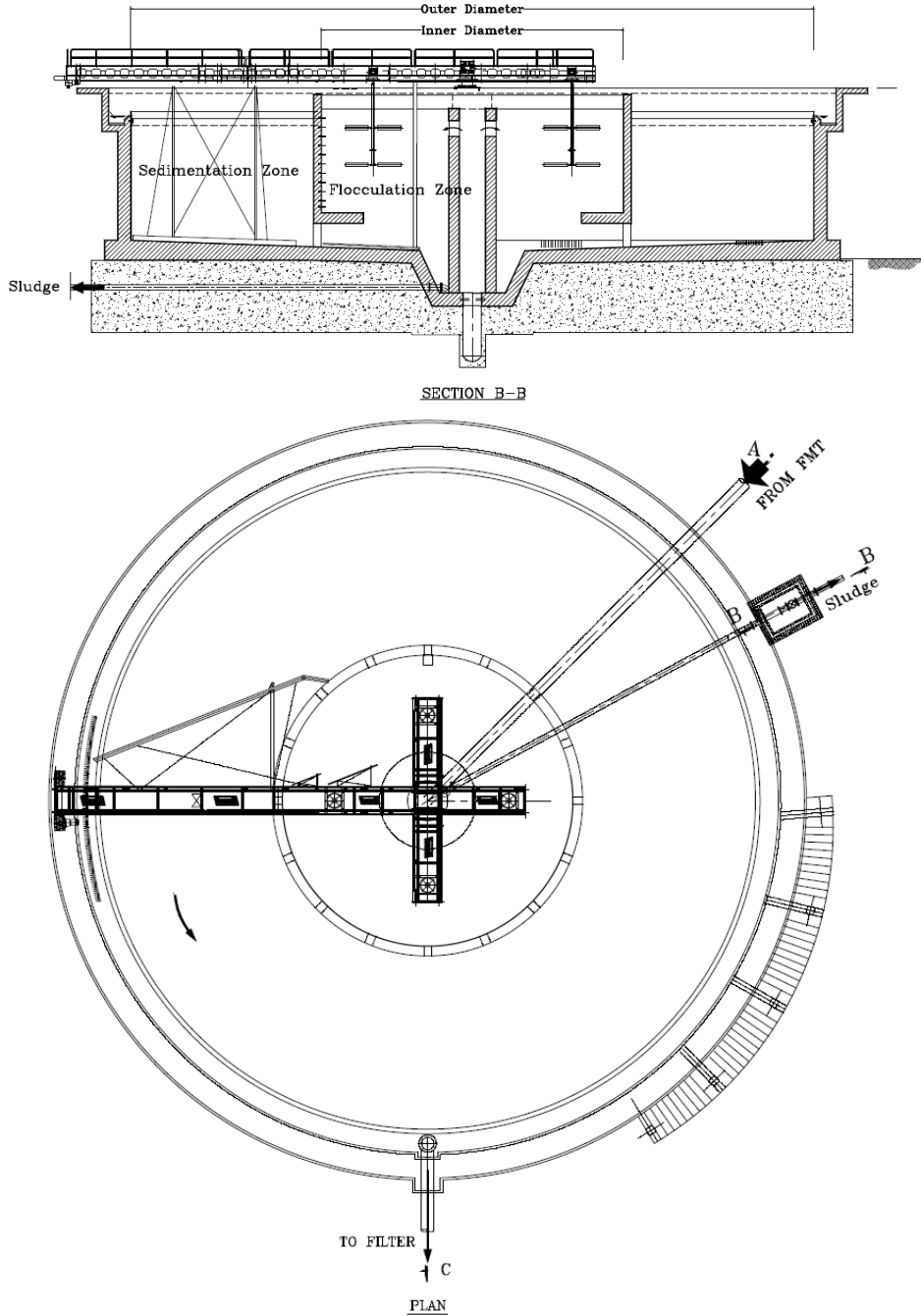
شكل (٢-٢٠) أحواض الترويب والتسيب العادية
