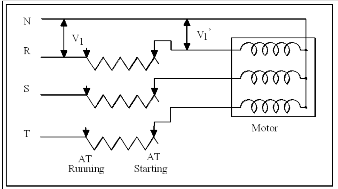
شكل (٤-١) البدء باستخدام مقاومات في العضو الثابت
