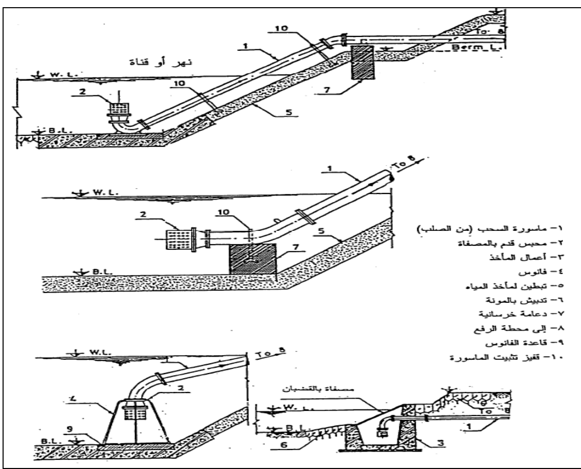
شكل (٢-٥) المآخذ المغمور (النموذج الثالث)
