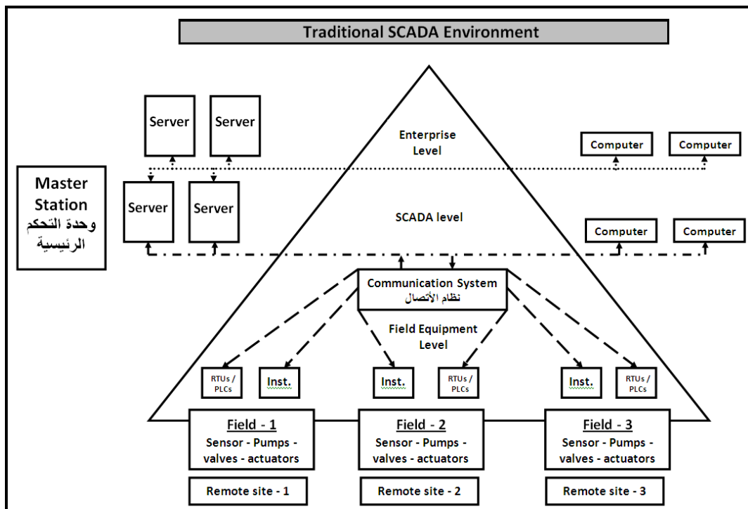
شكل (٤-١٦) بيئة تقليدية لنظام التحكم والمراقبة (SCADA)
