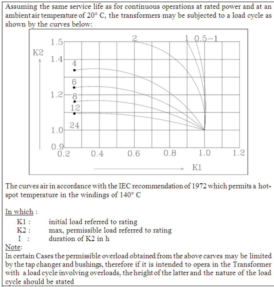
شكل (٨-٤) منحنى العلاقة بين k_1 ، k_2 عند القيم المختلفة لفترات التحميل t
