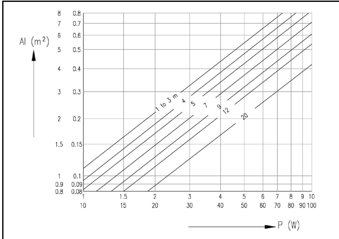
شكل (١٠-٤) نوموجرام تحديد مساحة فتحتي دخول وخروج الهواء
