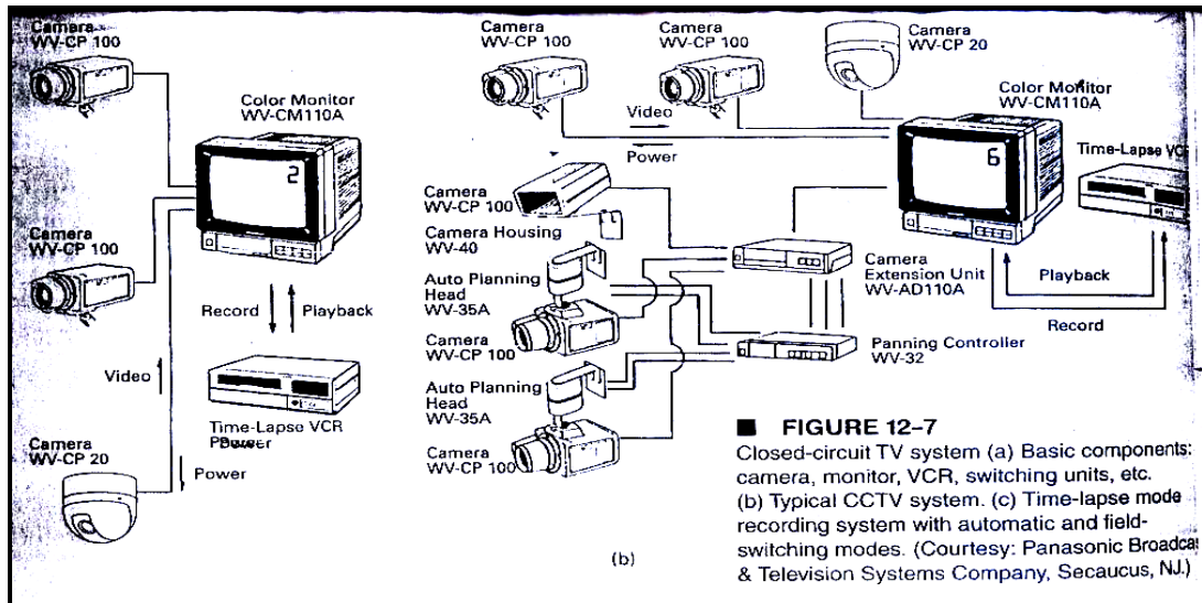
شكل (٤-١٨) نظم ودوائر المراقبة التلفزيونية (CCTV)
