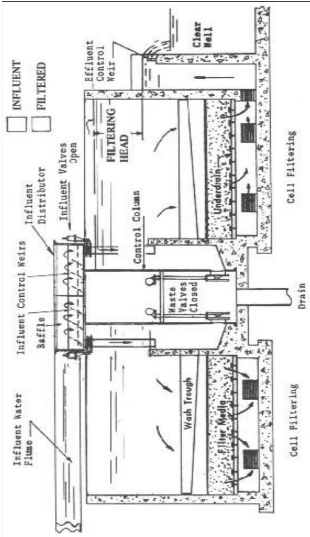
شكل (٢-٢٨) المرشحات الرملية السريعة (فوانى مركبة على بلاطة خرسانية لتجميع المياه المرشحة)
