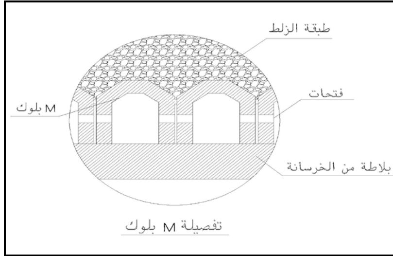
شكل (٢-٣١) شكل ال ( m بلوك ) التى تركيب بالمرشحات الرملية السريعة
