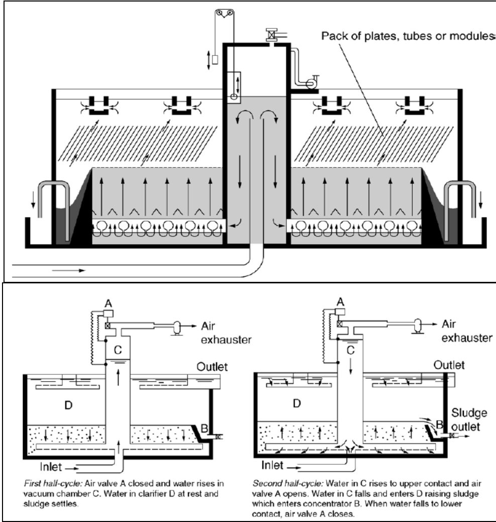
شكل (٢-٢٣) أحواض الترويق والترسيب السريعة أو ذات المعدل الفائق (Pulsator/Super Pulsator)
