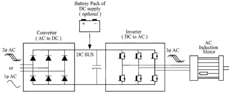
شكل (٤-٦) نظام قيادة لمحرك تآثيرى ثلاثى الطور
