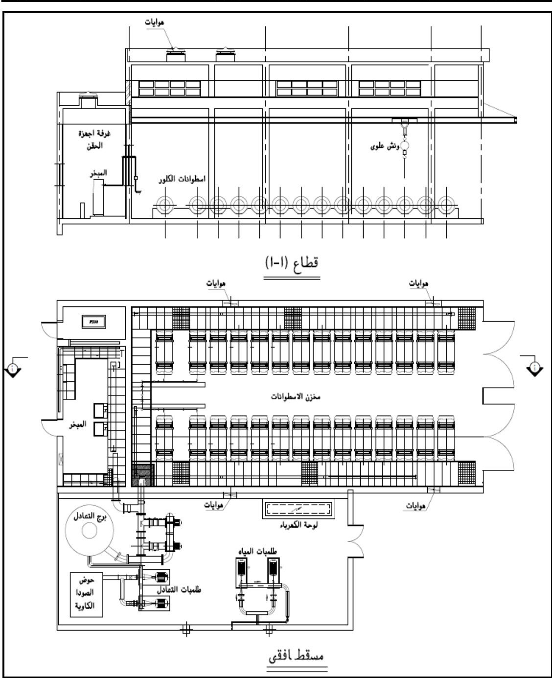
شكل (٢-٣٧) عنبر إضافة الكلور
