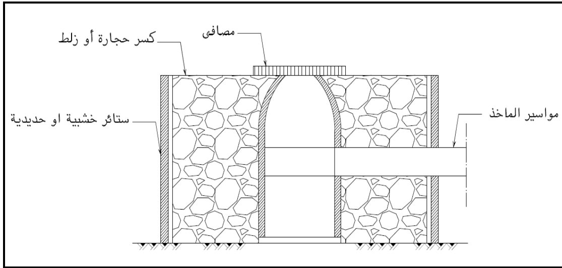
شكل (٢-٣) المآخذ المغمور (النموذج الأول)
