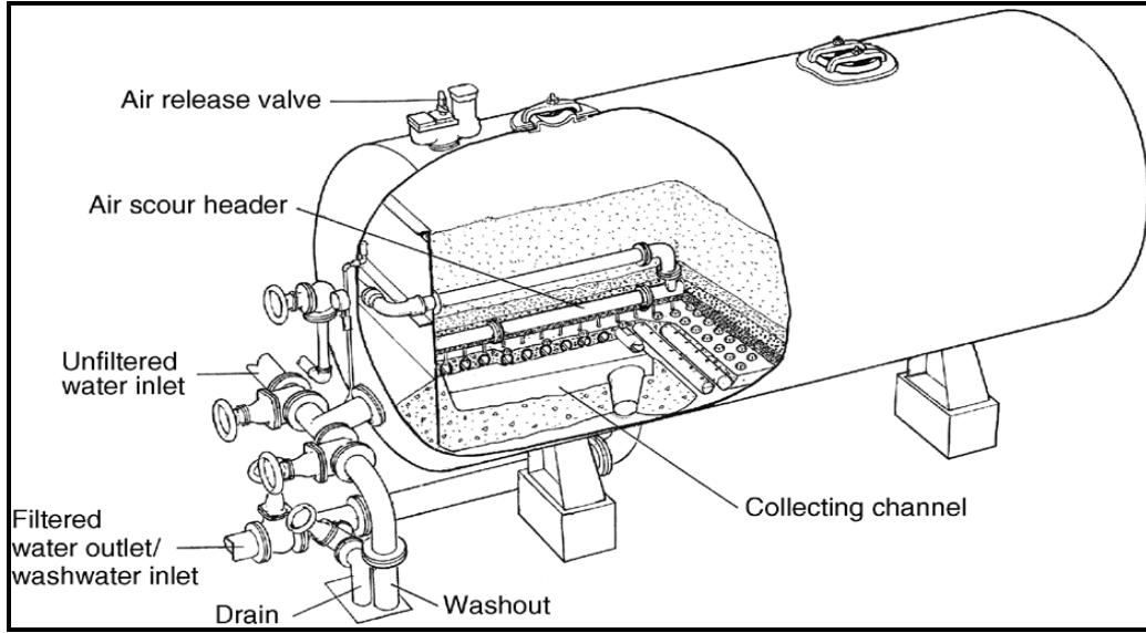
شكل (٢-٣٢) تفاصيل مرشح ضغط افقى
