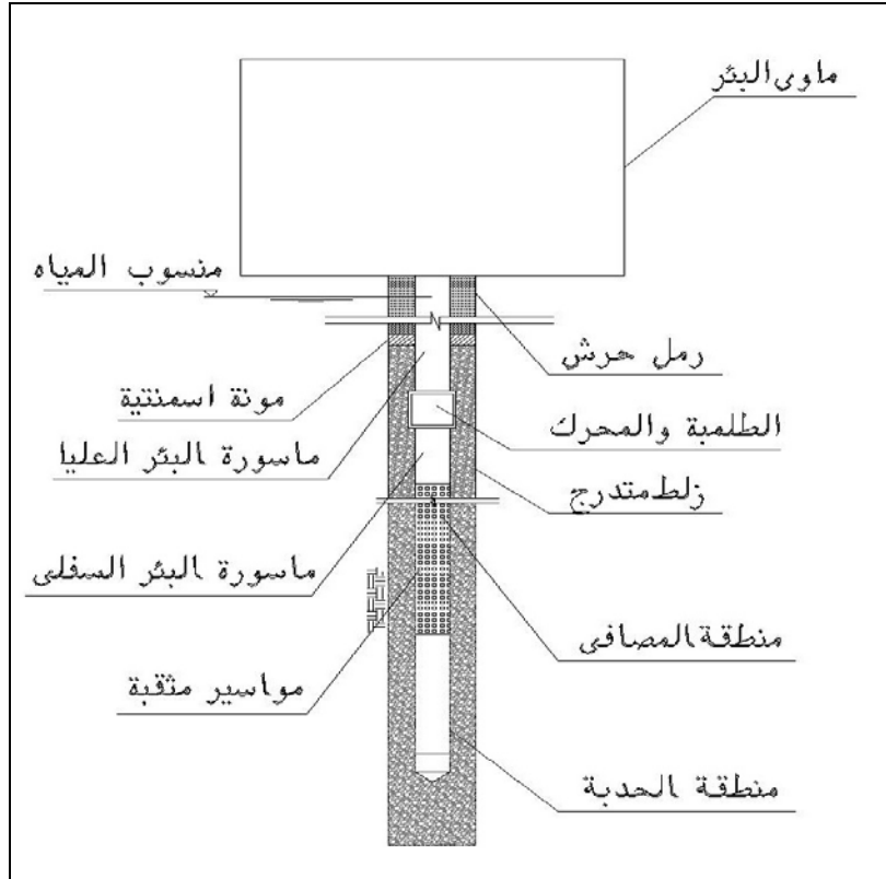
شكل (٢-٣٨) مكونات البئر الجوفى
