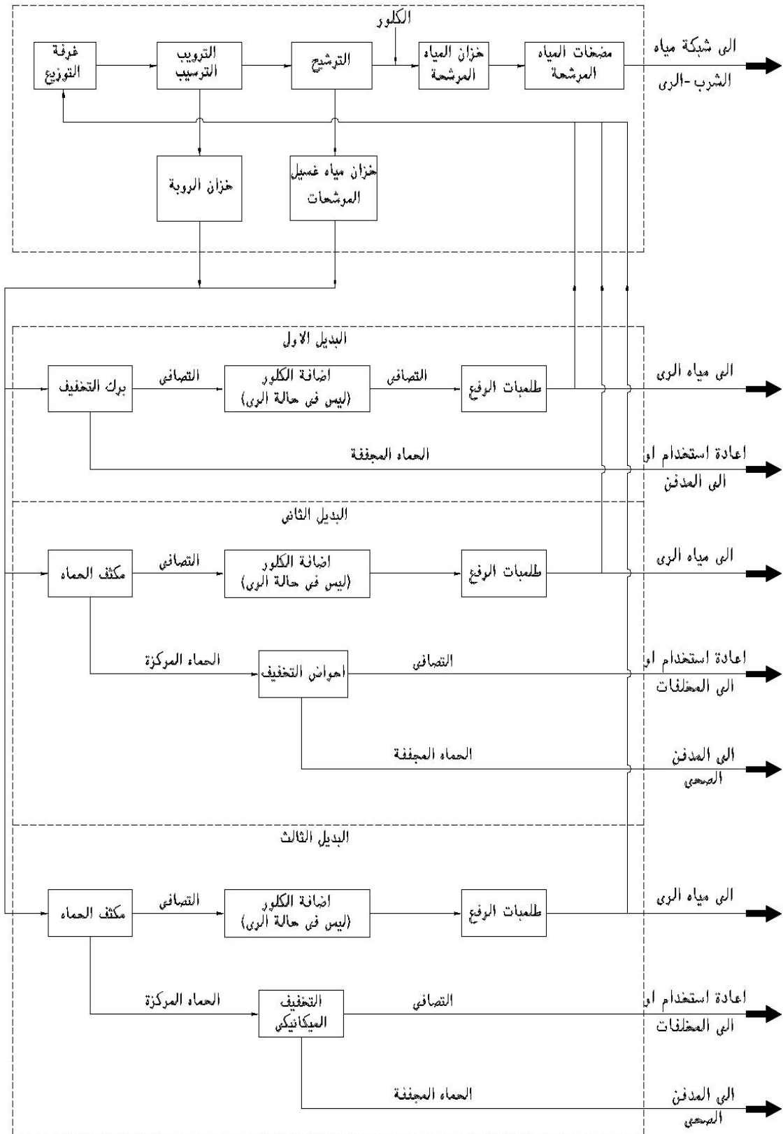
شكل (٢-٤٠) مراحل معالجة الروبة
