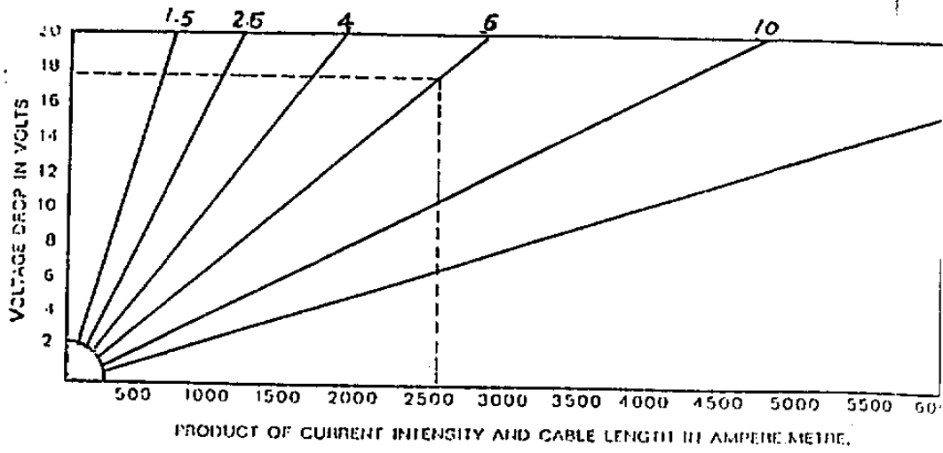
شكل (٤-١٢) نوموجرام حساب التنزيل في الجهد للكابلات ثنائية القطب لإمرار التيار ذو الوجه الواحد عند معامل قدرة واحد صحيح.
