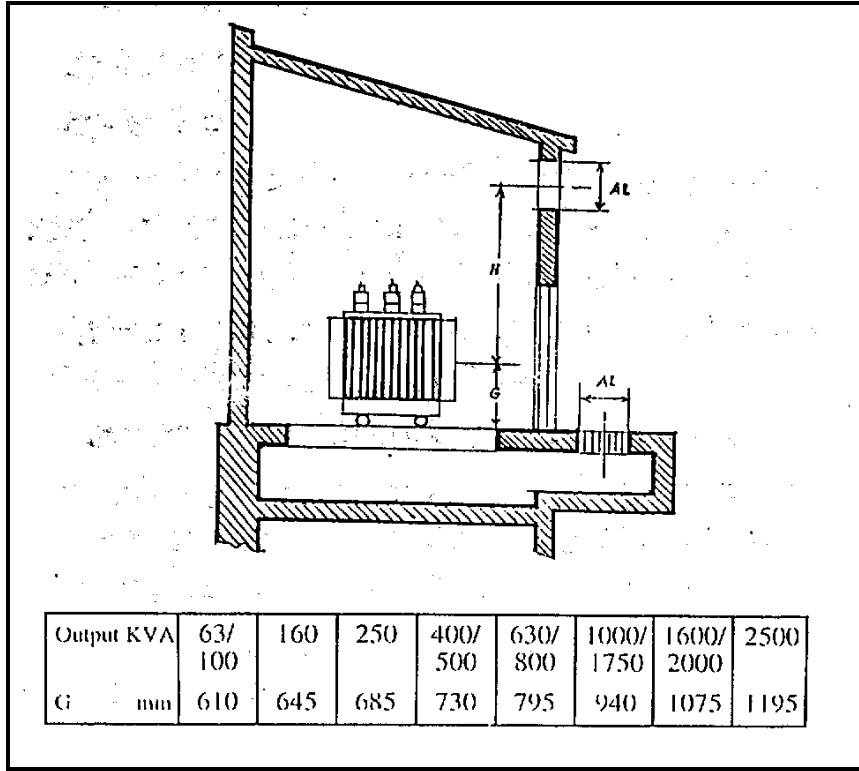
شكل (١١-٤) تركيب المحولات في مأوى مغلق
