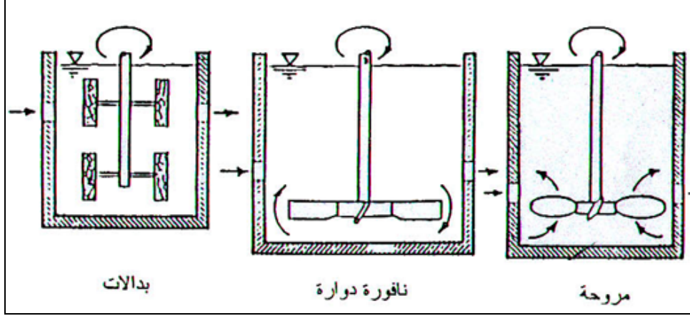
شكل (١١-٢) طرق الخلط الميكانيكى السريع
