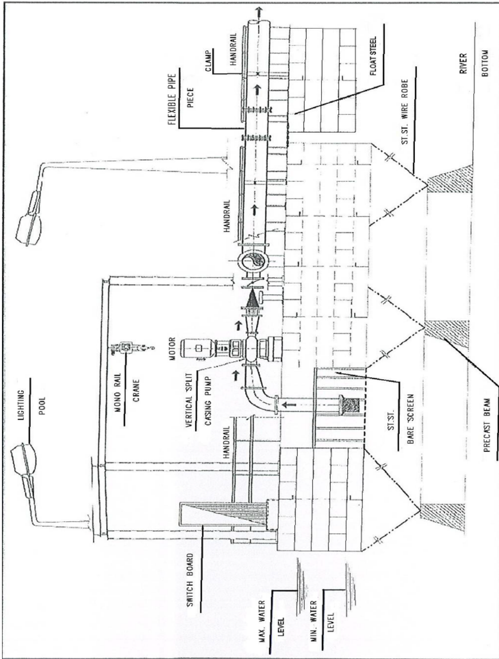
شكل ( ٧-٢ ) المآخذ العائم
