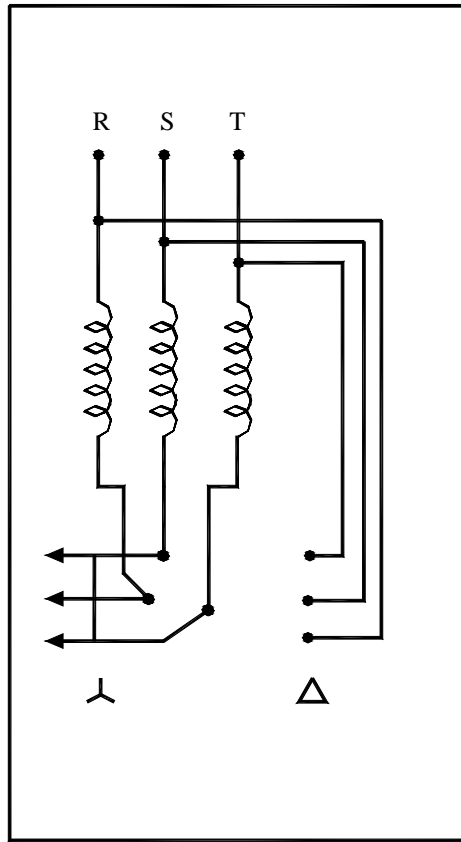
شكل (٤-٤) البدء باستخدام سكينه نجمة / دلتا
