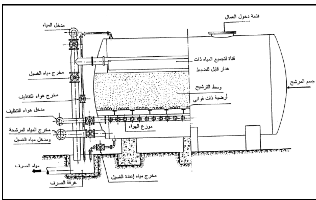
شكل (٢-٤٣) تفاصيل مرشح ضغط أفقى
